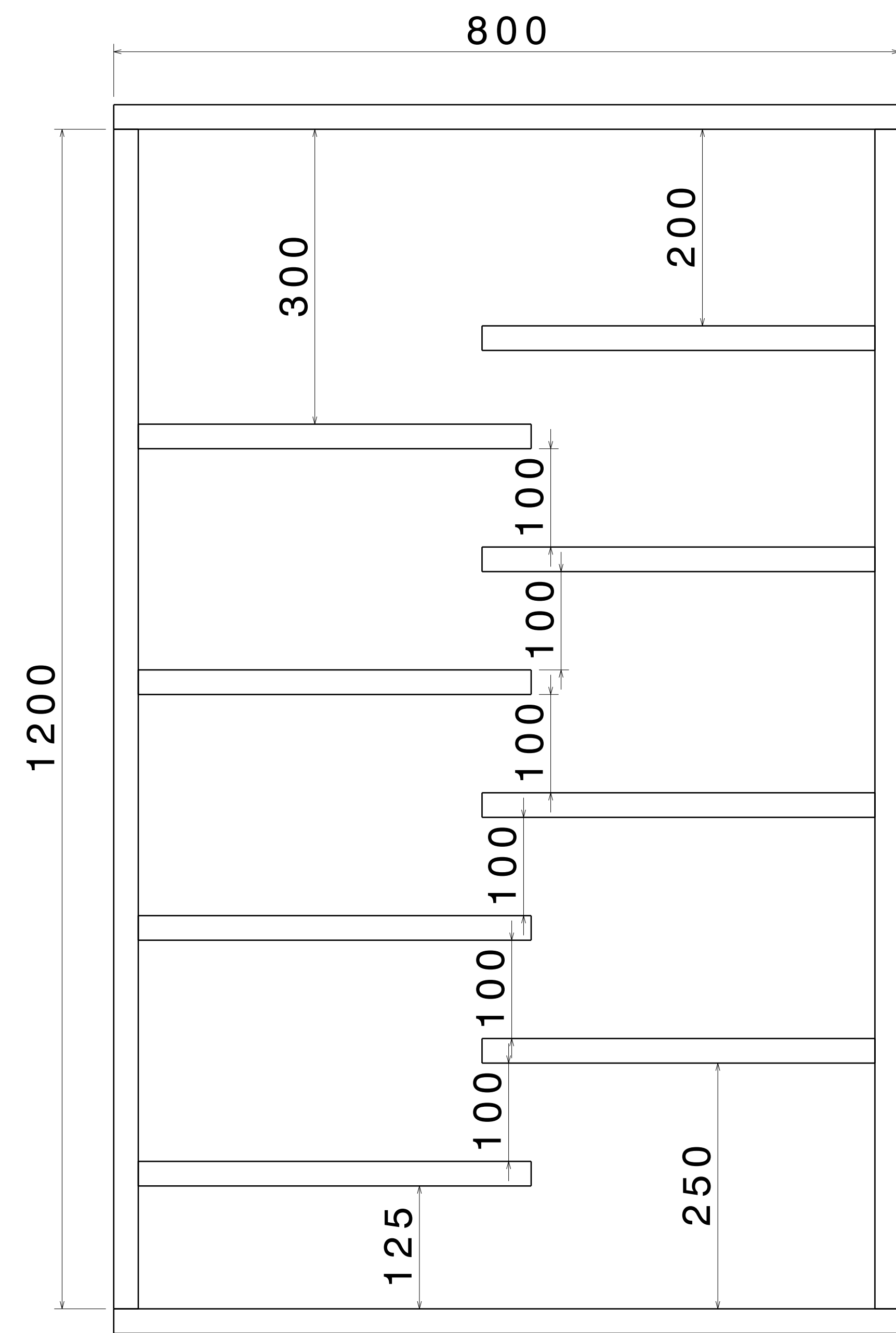
Front view Scale: 1:4
