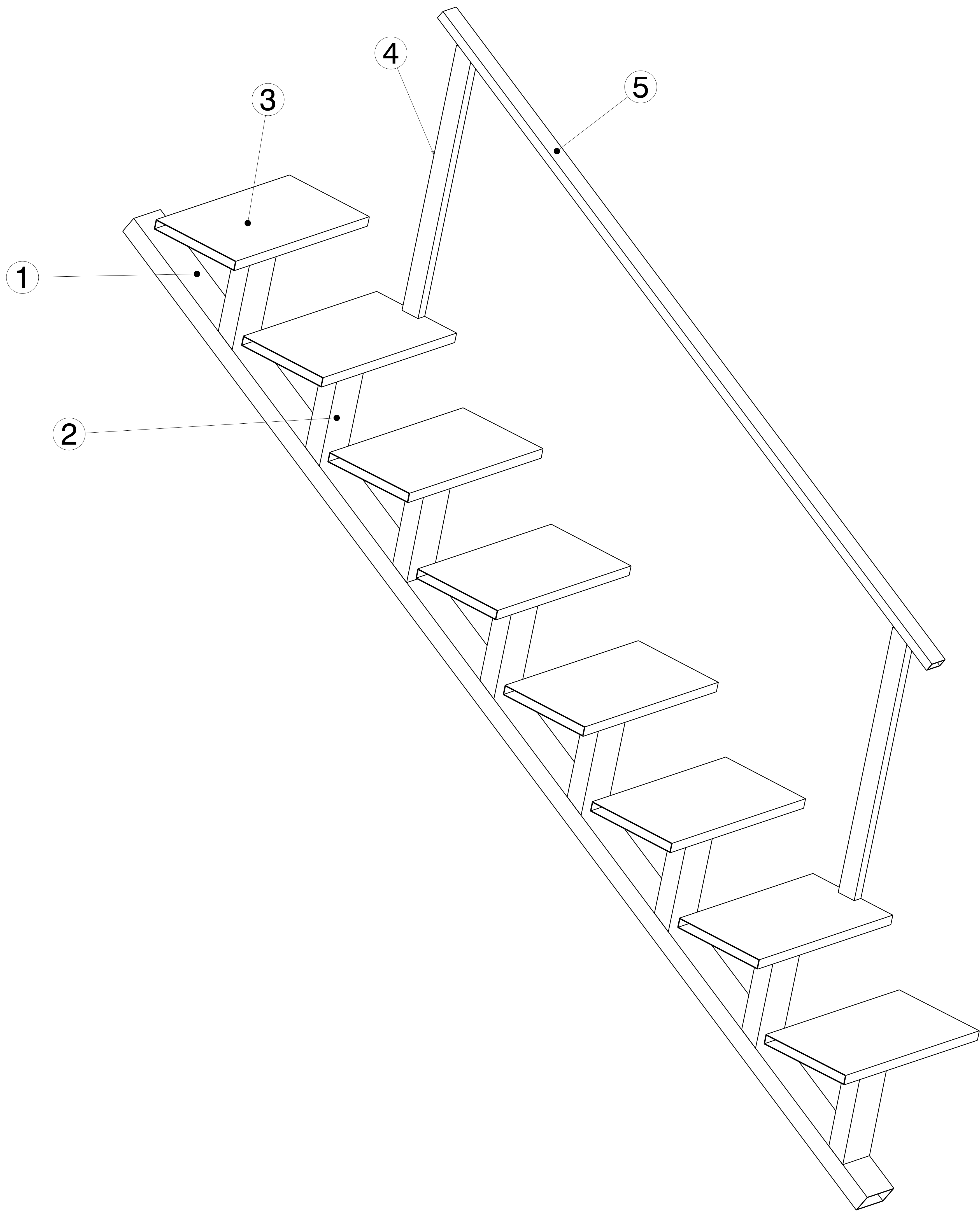
Isometric view Scale: 1:5
