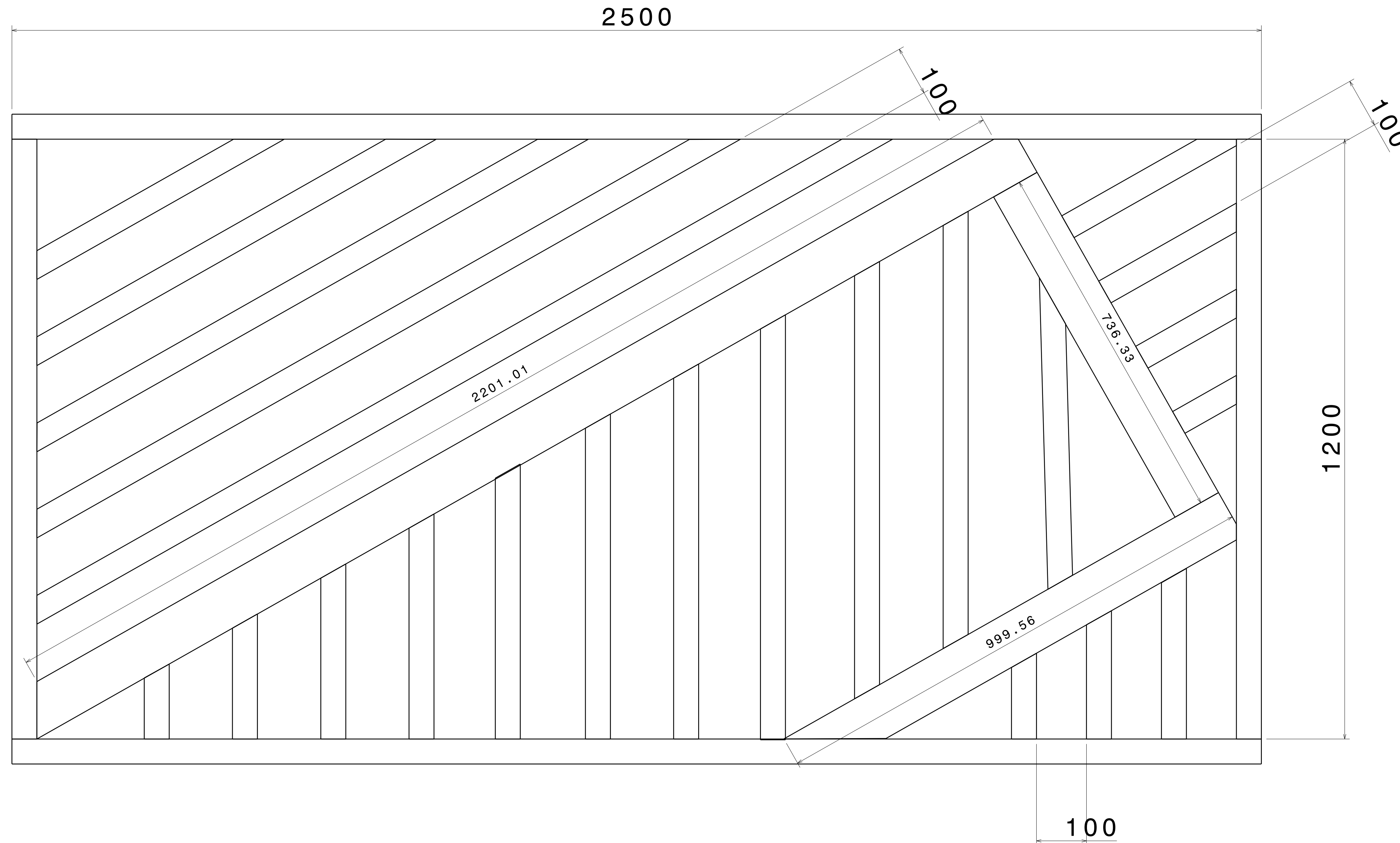
Front view Scale: 1:5
