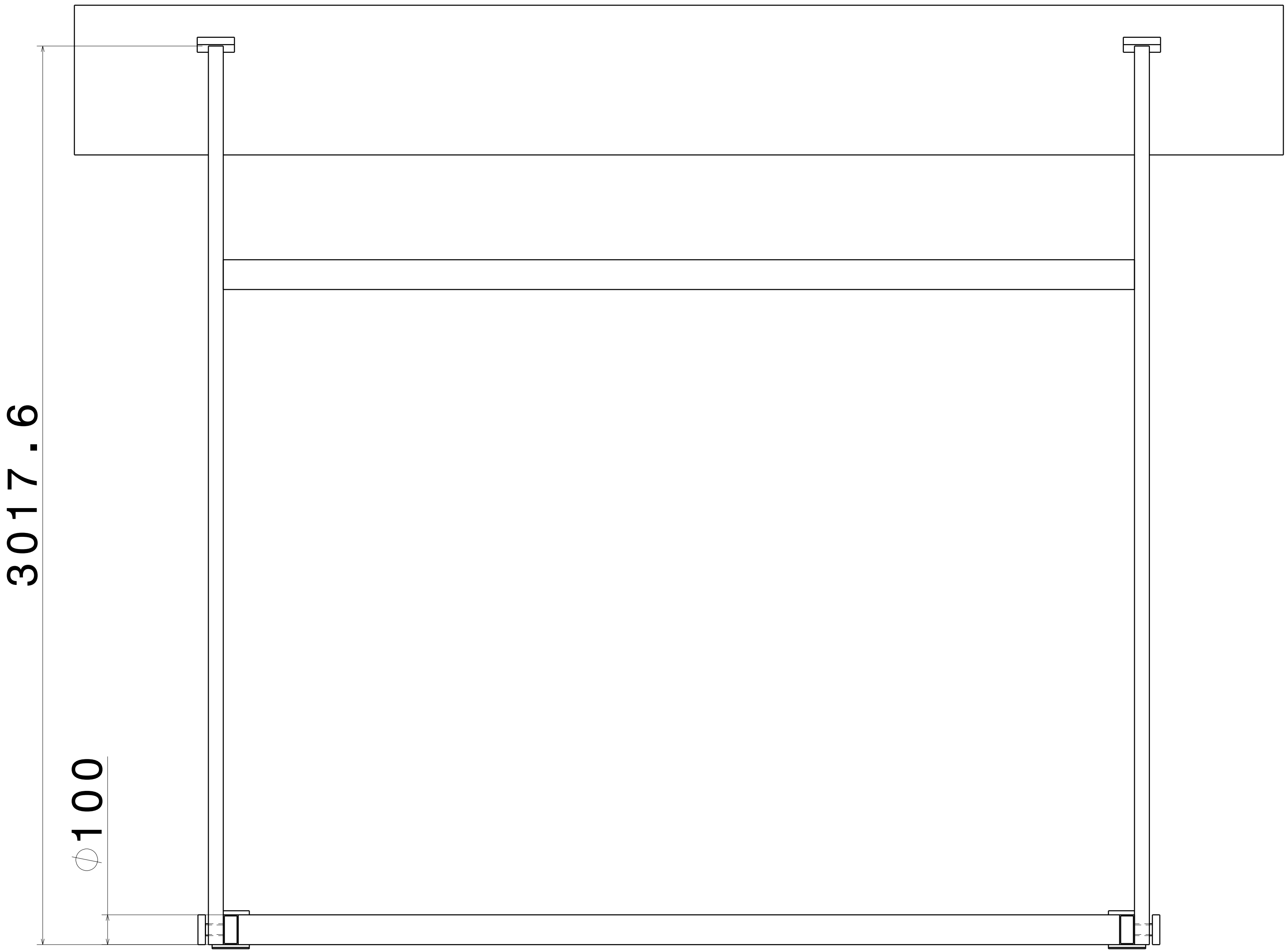
TOP VIEW SCALE: 1:10
