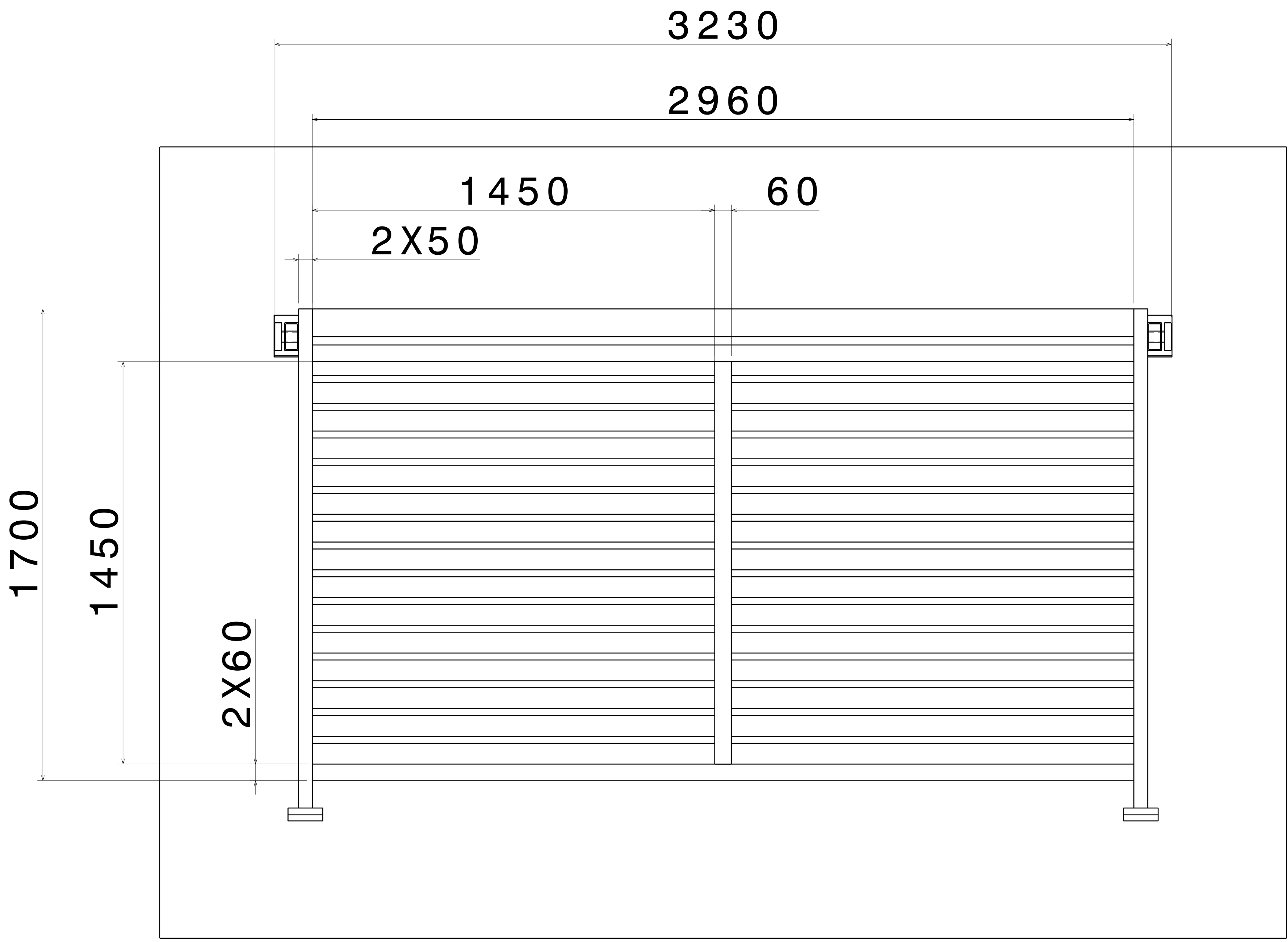
TOP VIEW SCALE: 1:10
