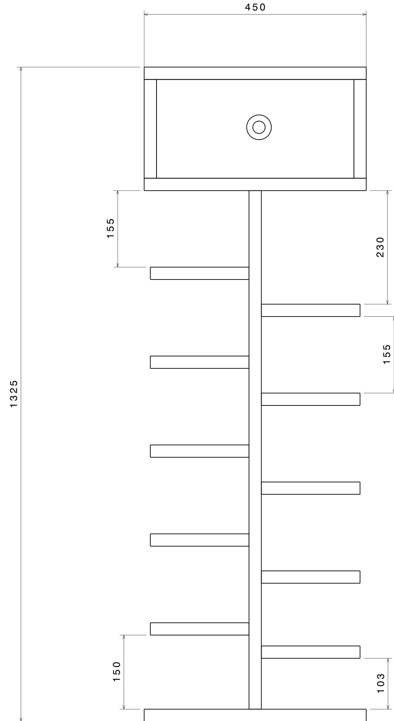
Front view Scale: 1:4
