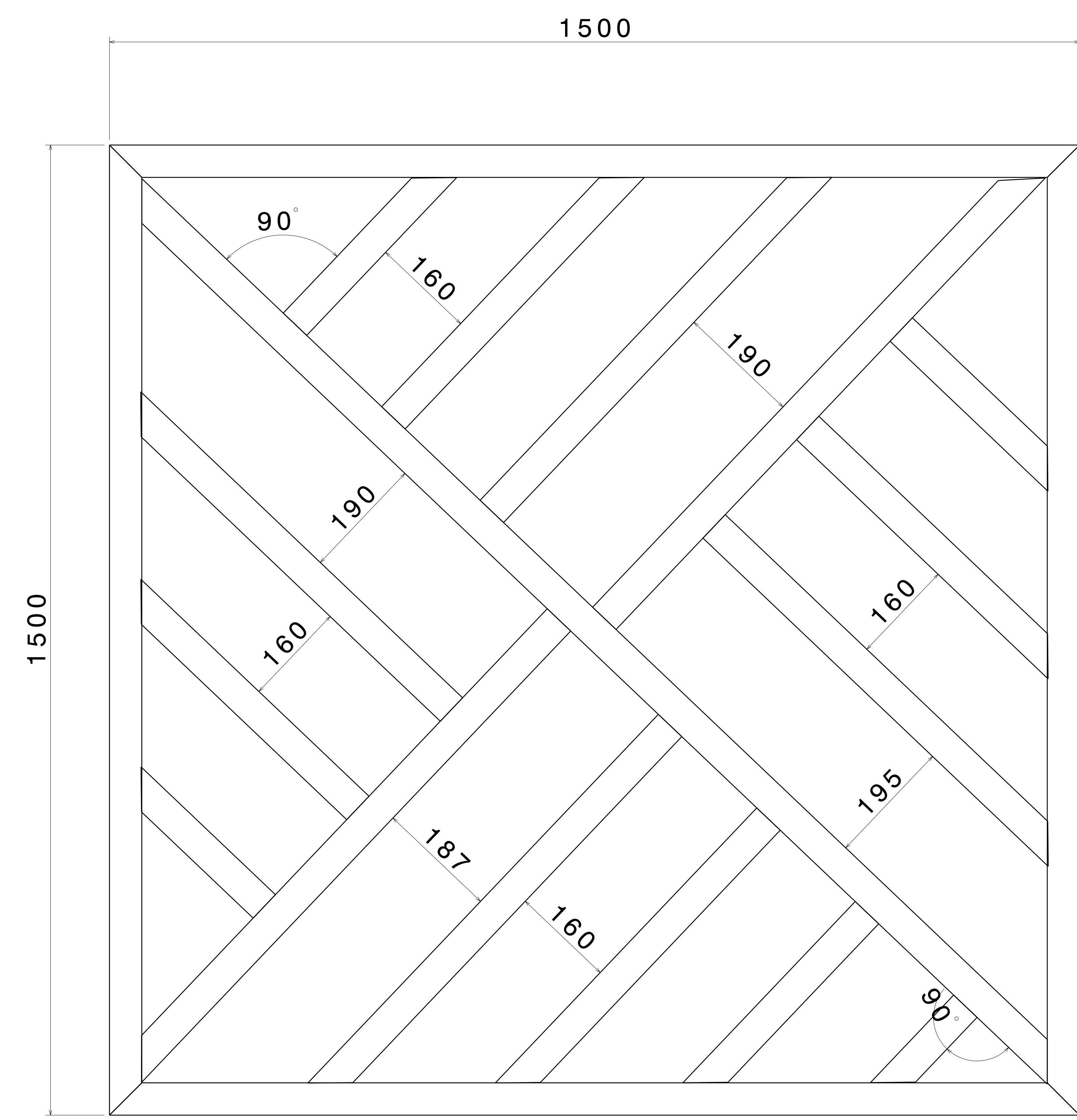
Front view Scale: 1:4
