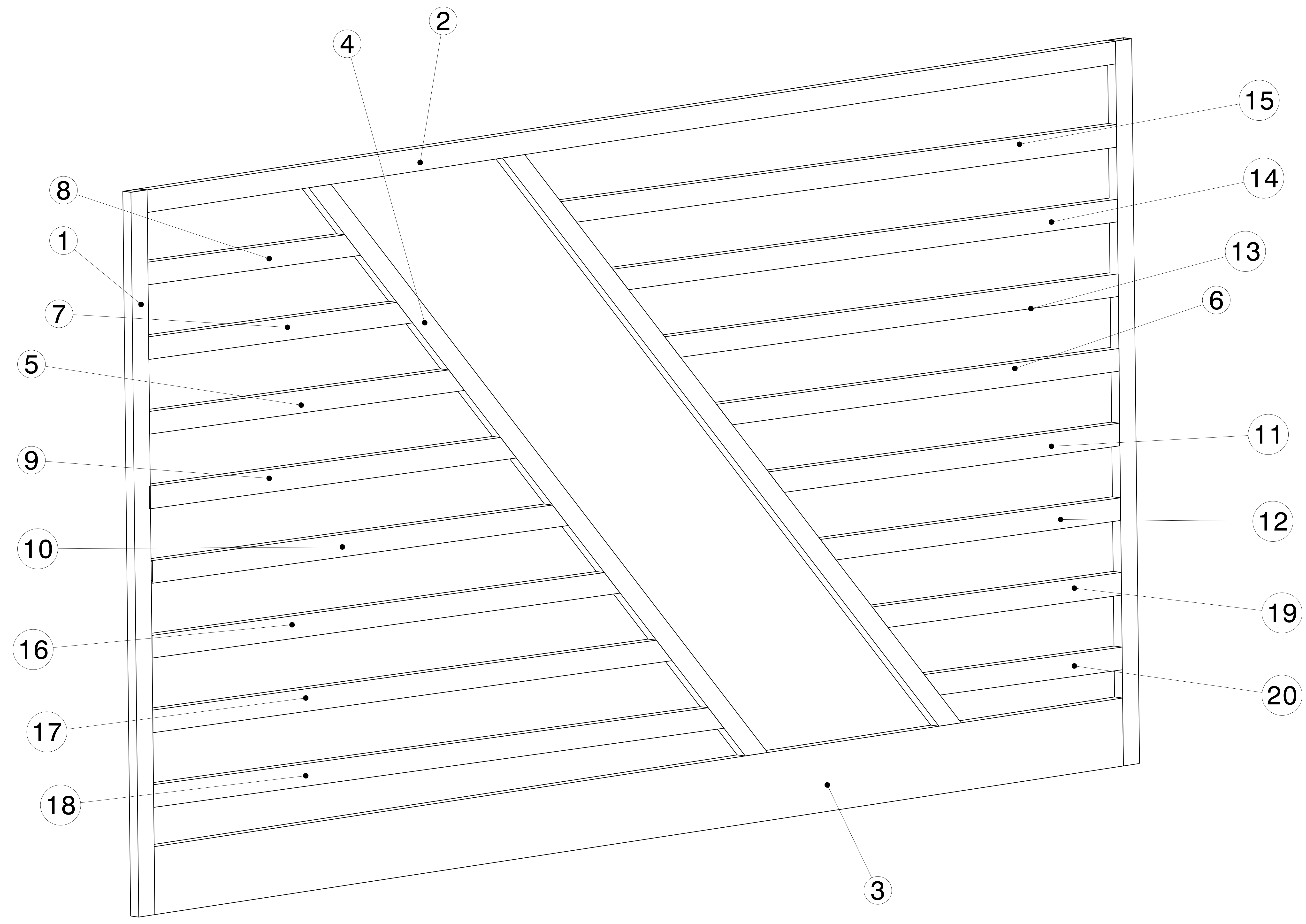
Isometric view Scale: 1:4
