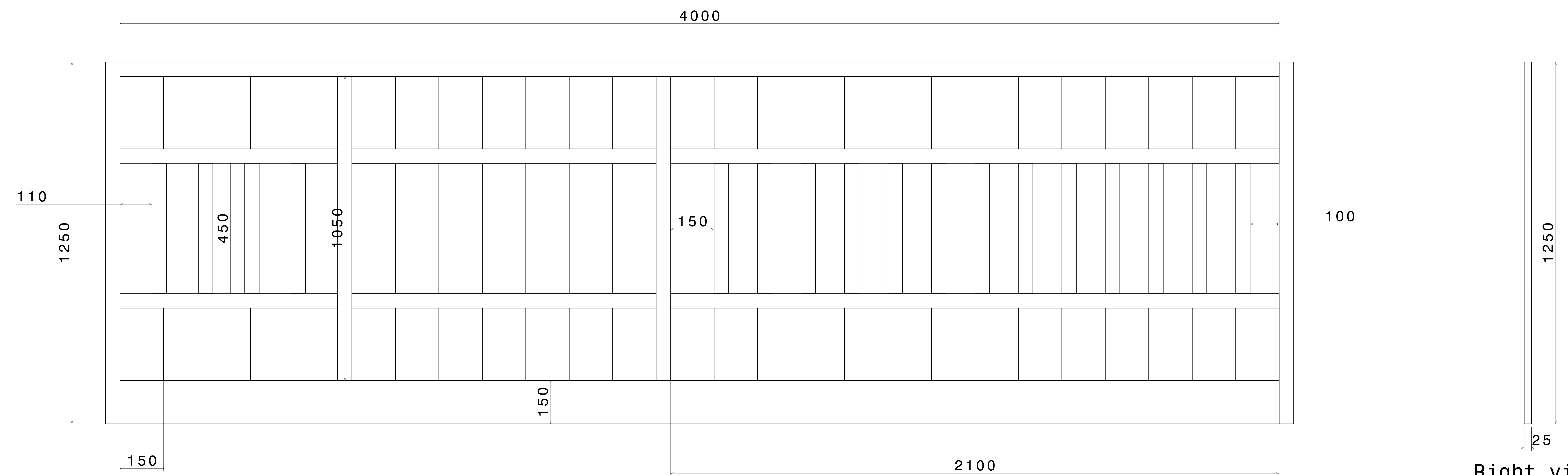
Front view Scale: 1:5
