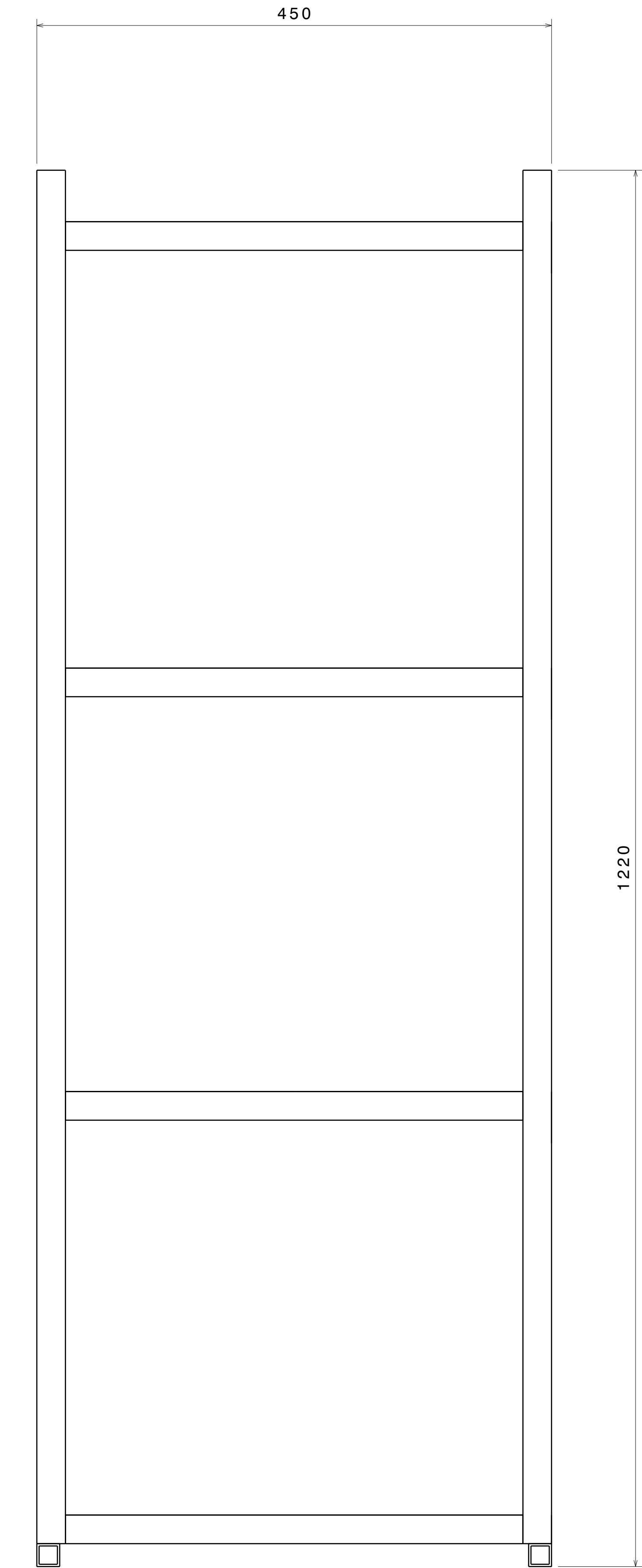
Right view Scale: 7:20
