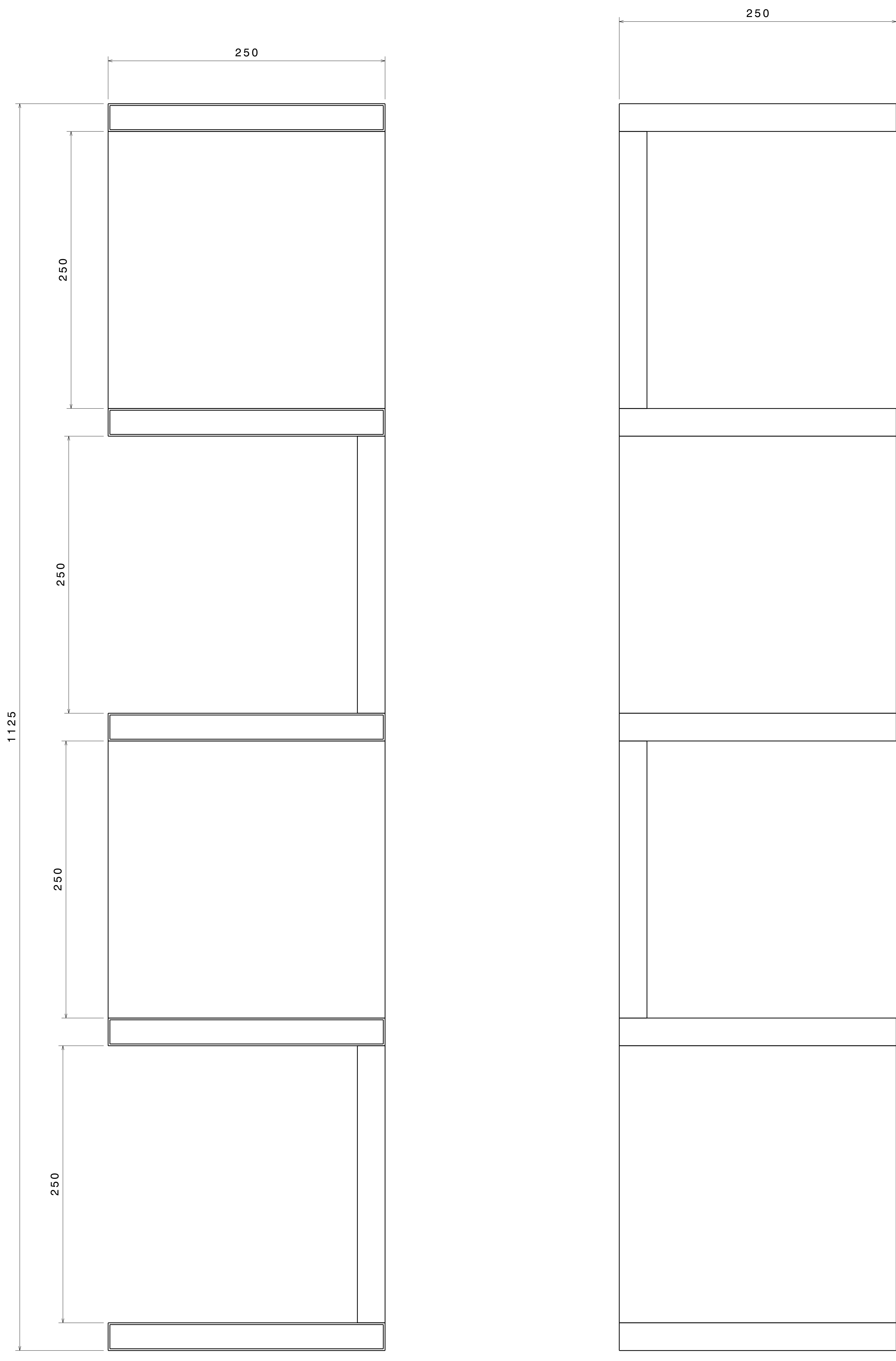
Right view Scale: 1:2
