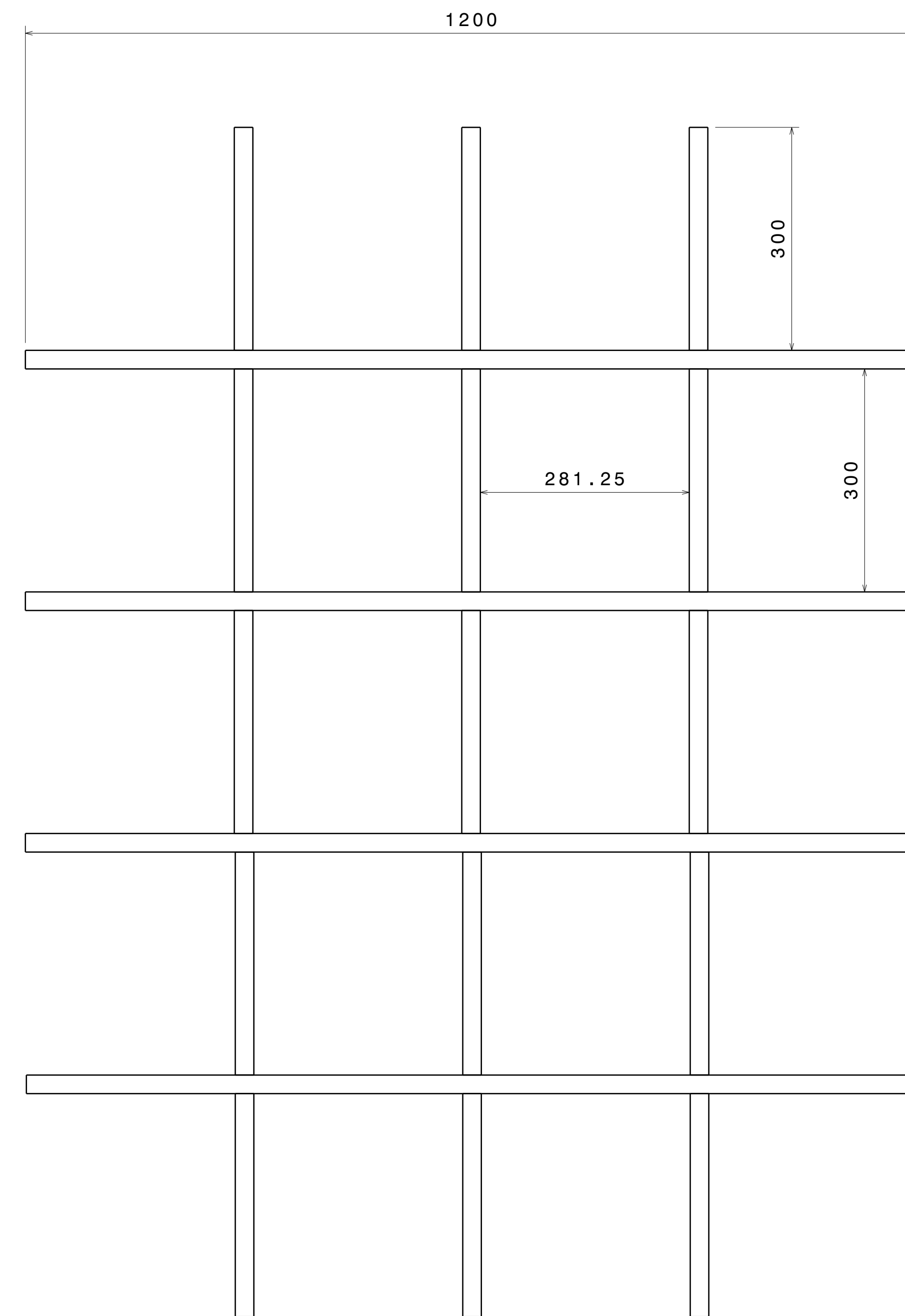
Front view Scale: 1:5
