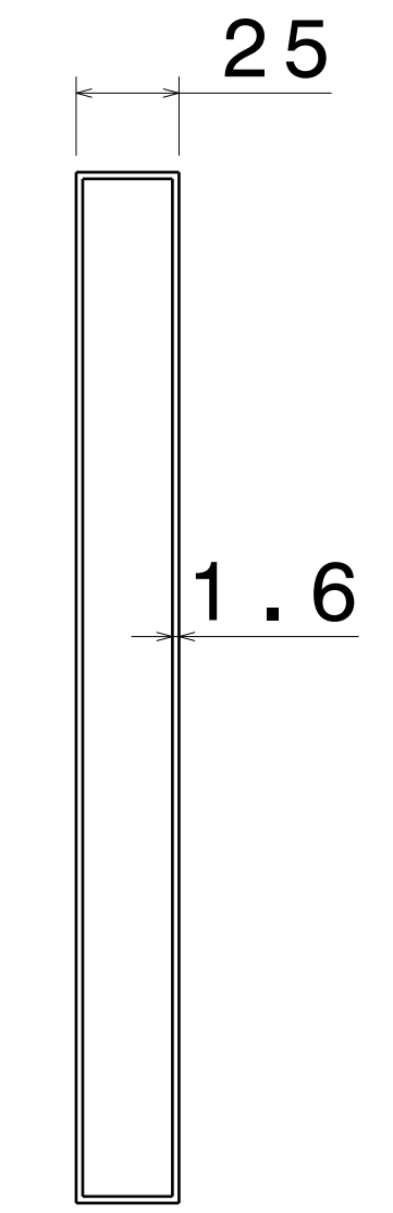
Right view Scale: 1:2
