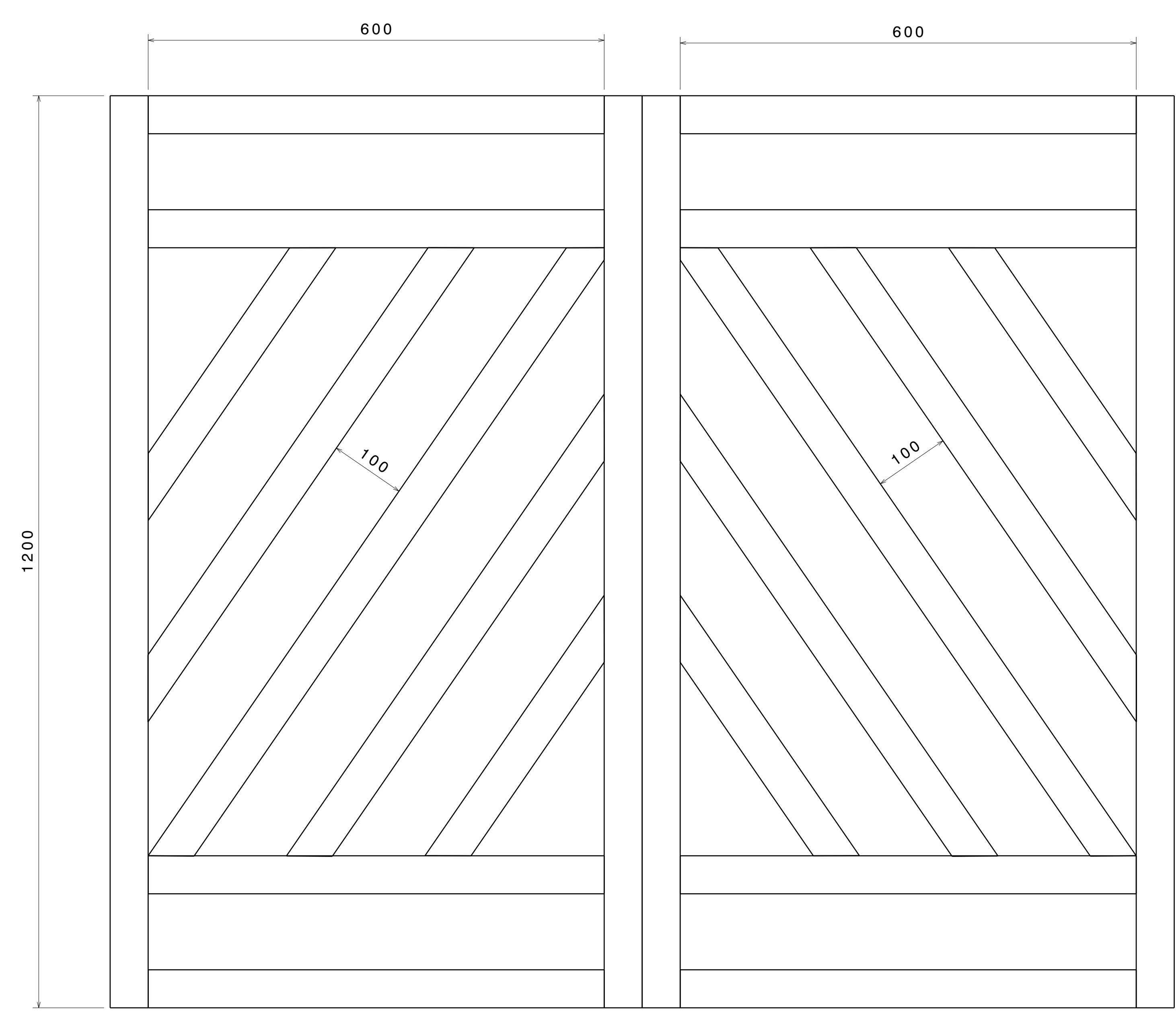
Front view Scale: 1:4
