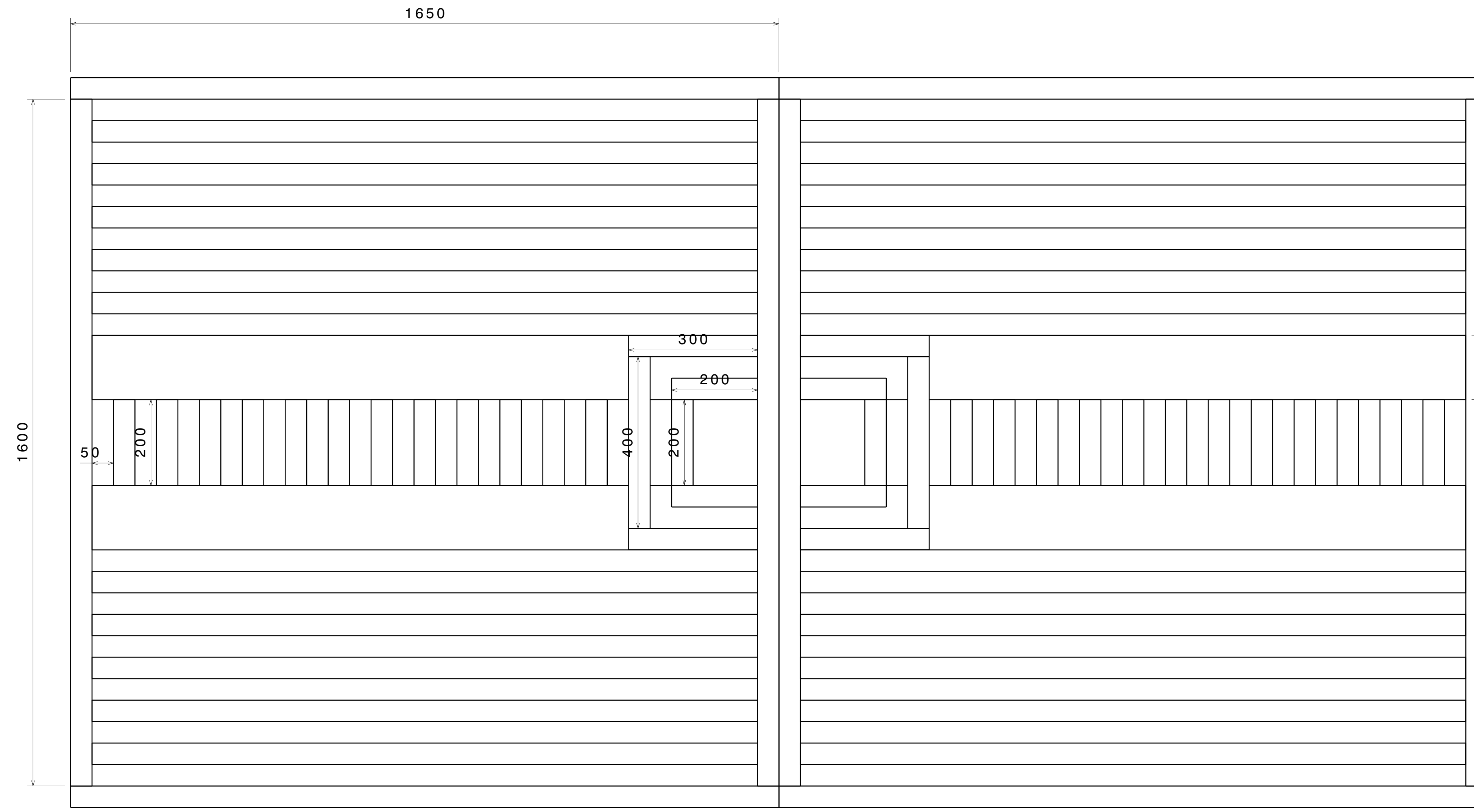
Front view Scale: 3:20
