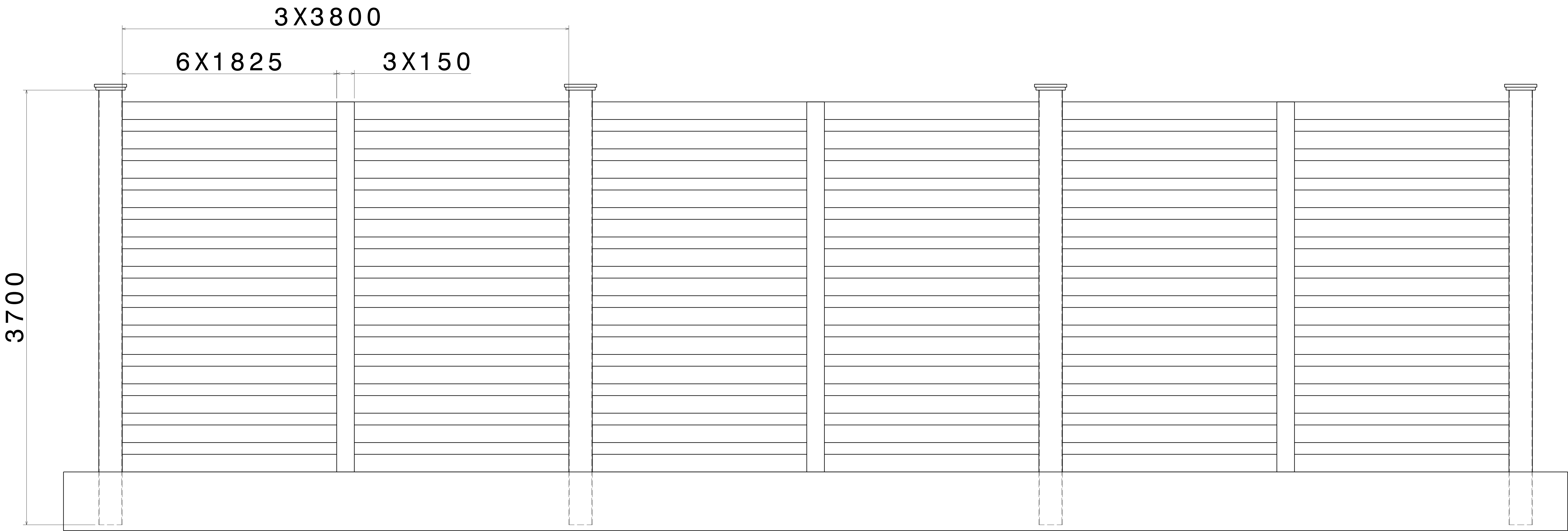
FRONT VIEW SCALE: 1:15
