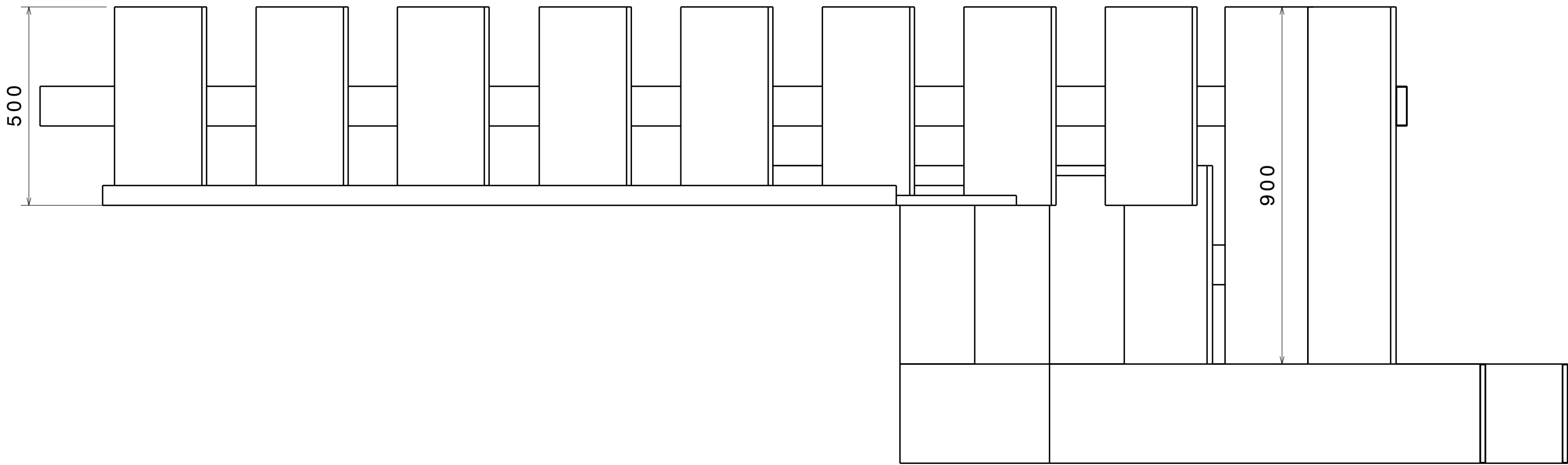
Top view Scale: 1:10
