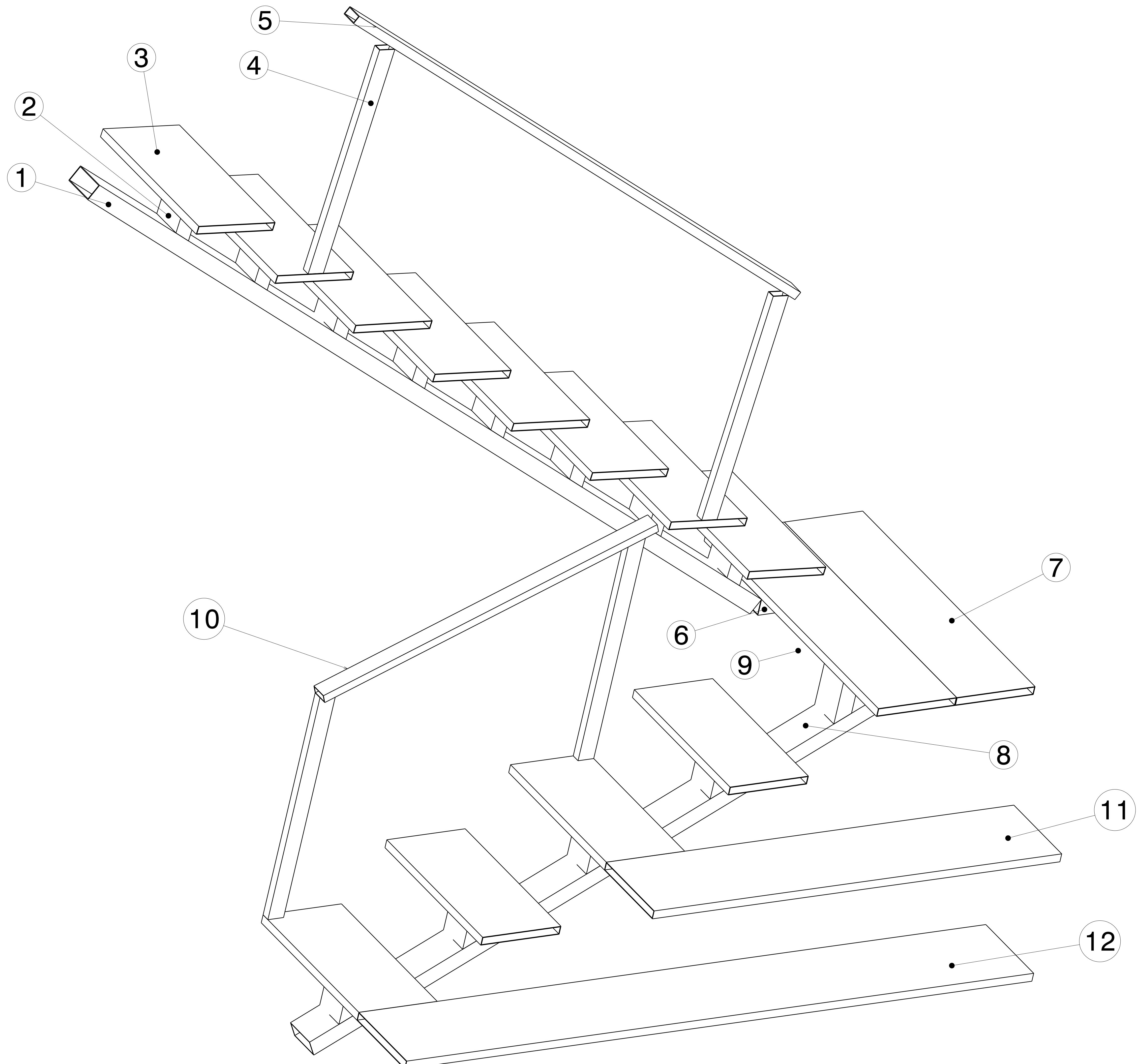
Isometric view Scale: 1:5
