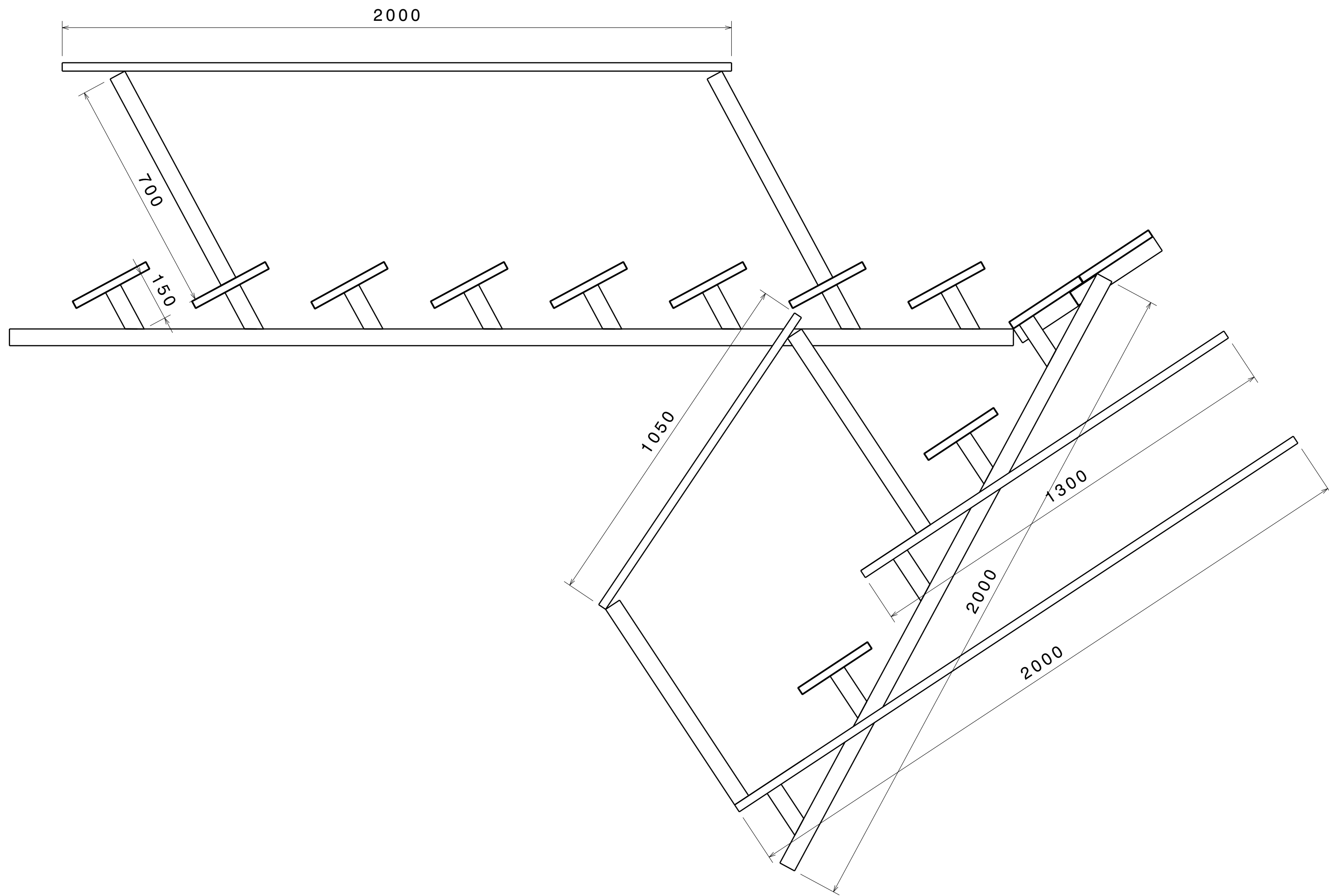
Front view Scale: 1:10
