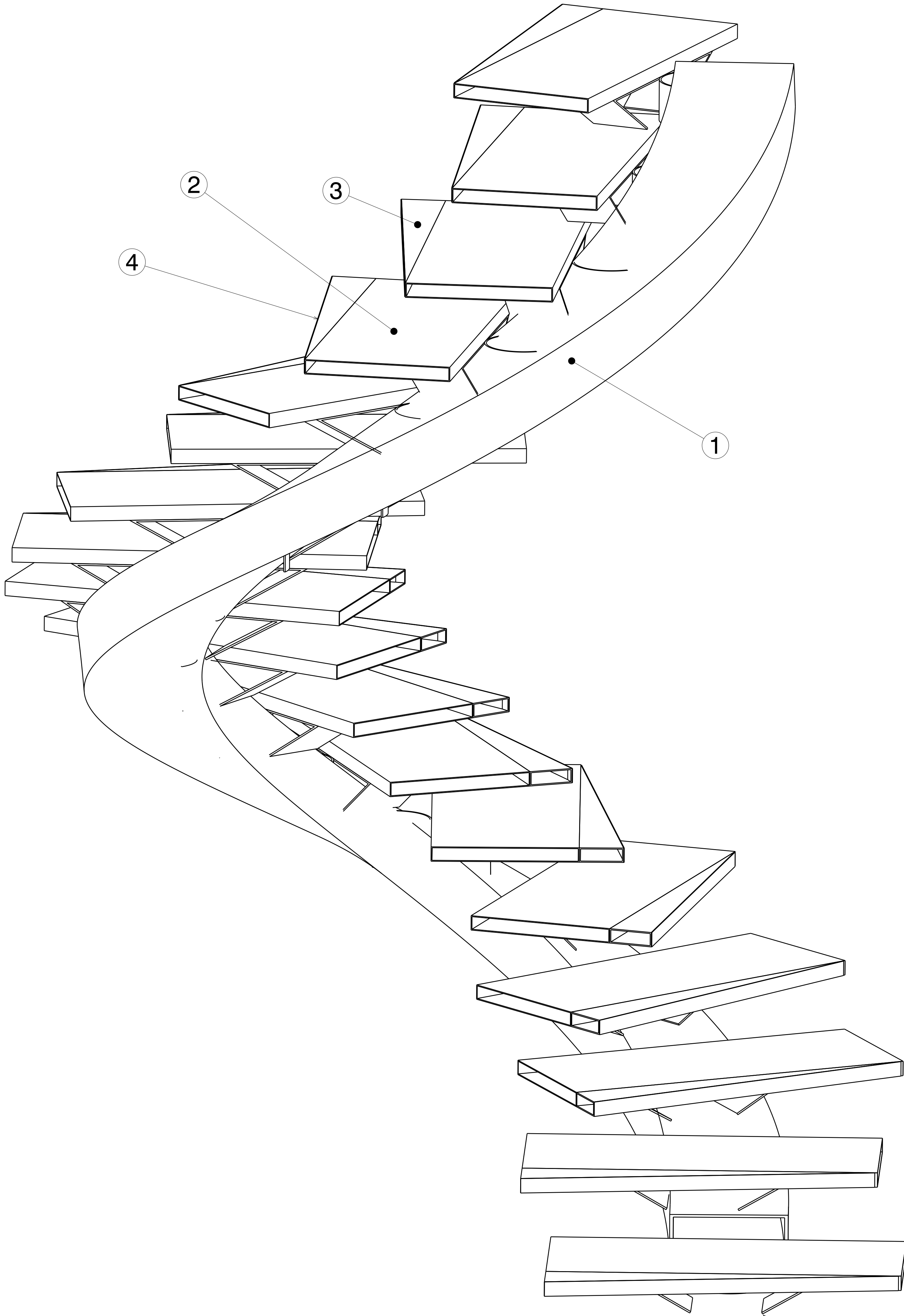
Isometric view Scale: 1:4
