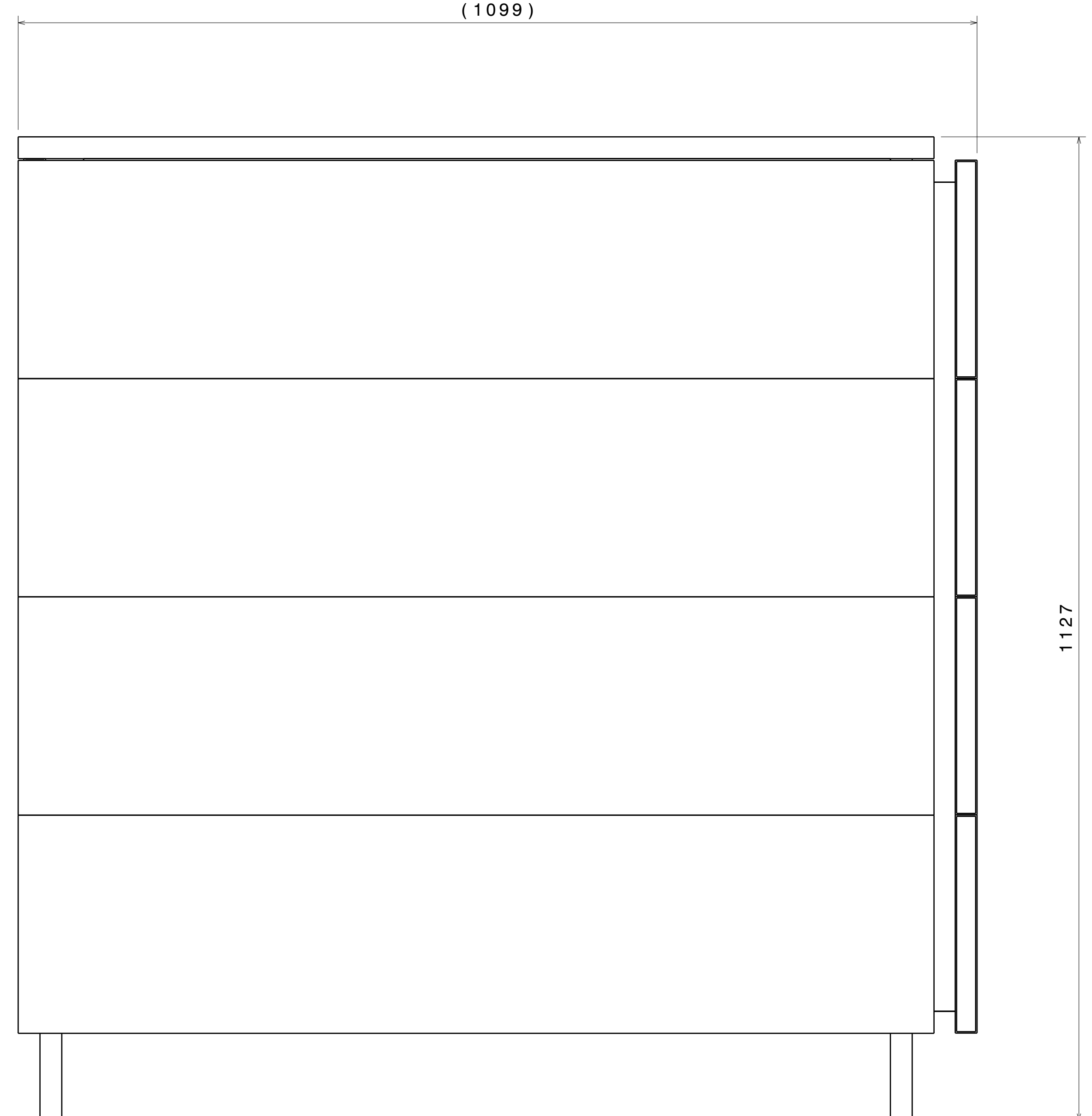
Front view Scale: 1:4
