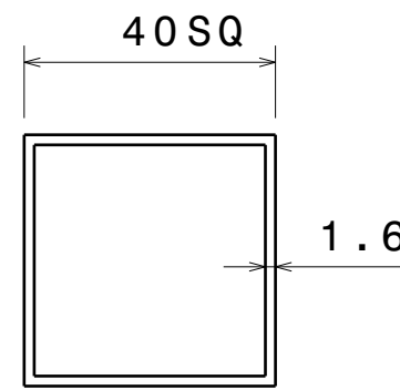
Top view Scale: 3:4
