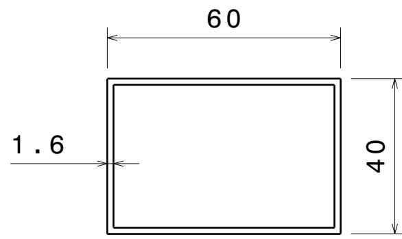
Top view[4] Scale: 3:4
