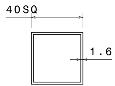
Top view[2] Scale: 3:5
