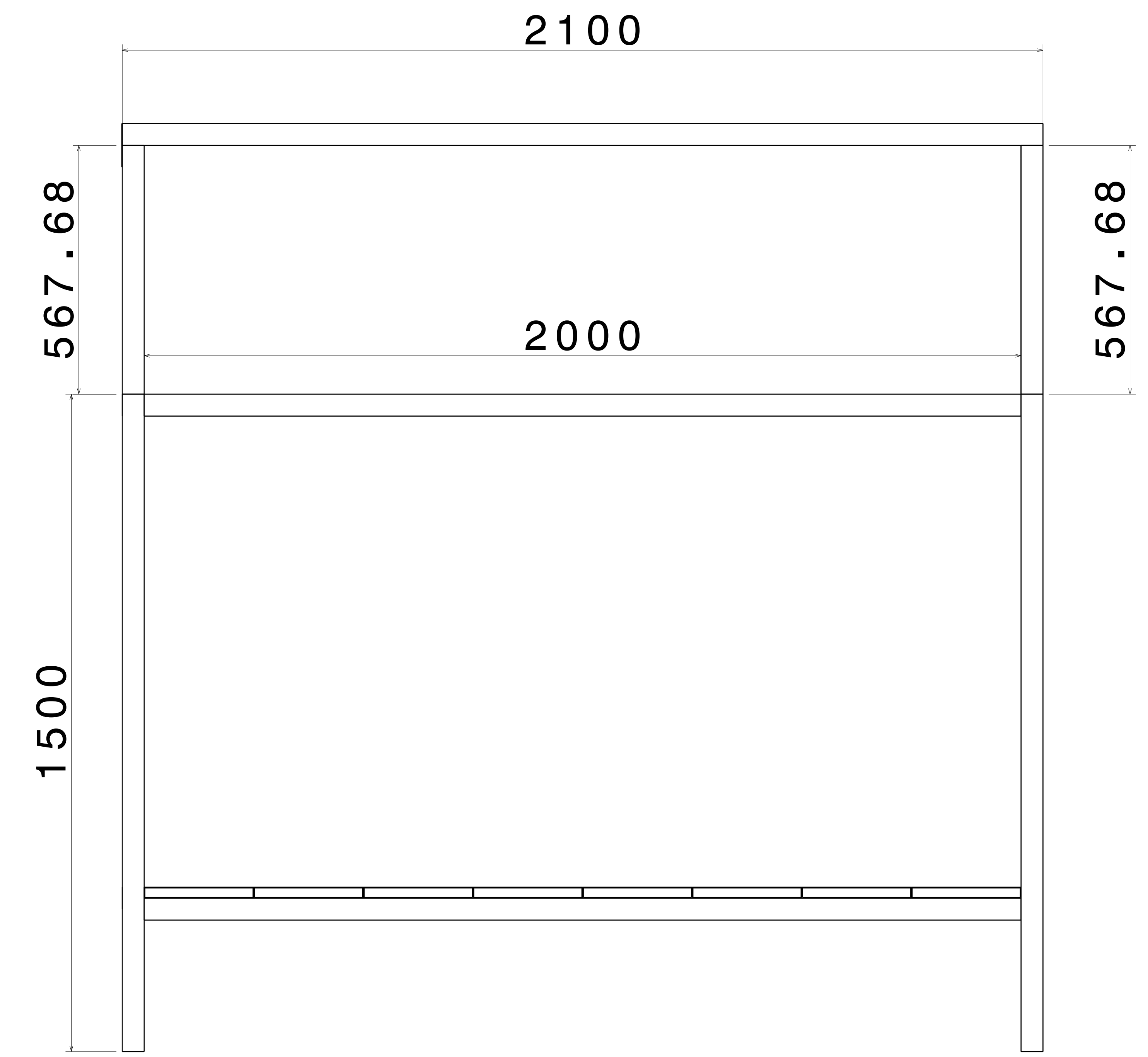
Front view Scale: 3:20
