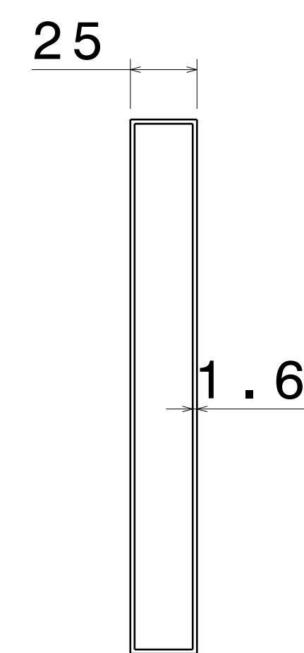
Right view Scale: 1:2
