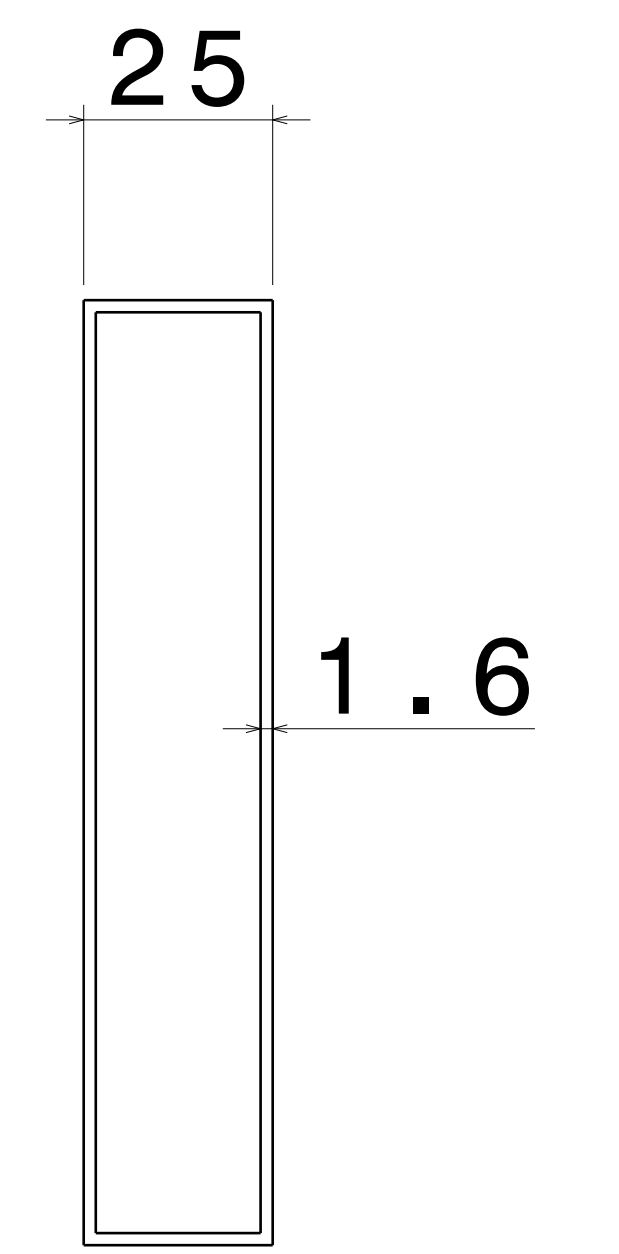
Right view Scale: 1:1
