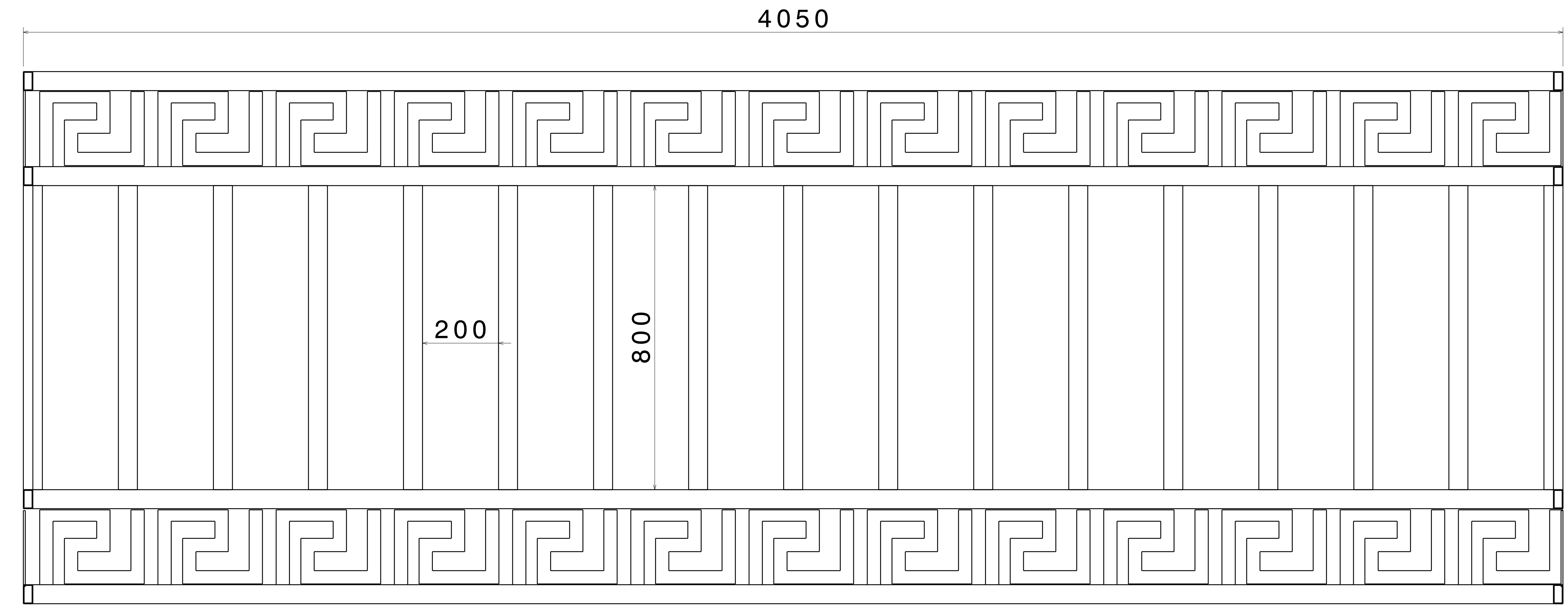
Front view Scale: 3:20
