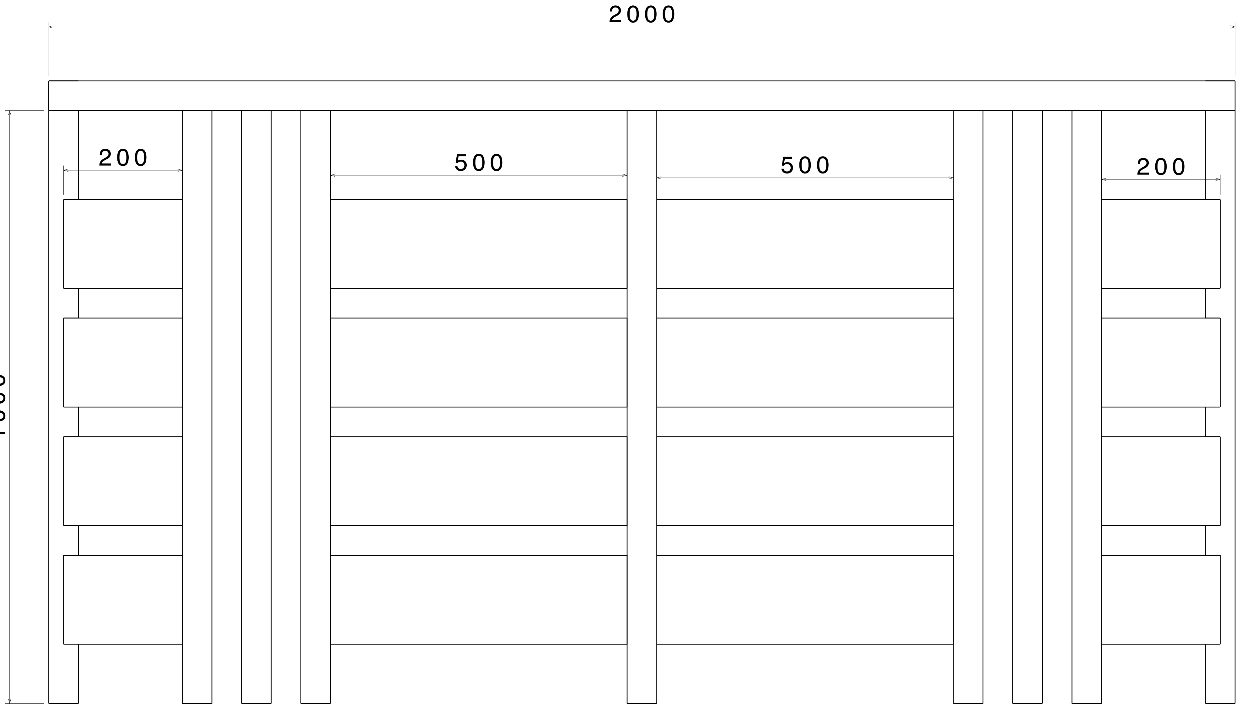
Front view Scale: 1:4
