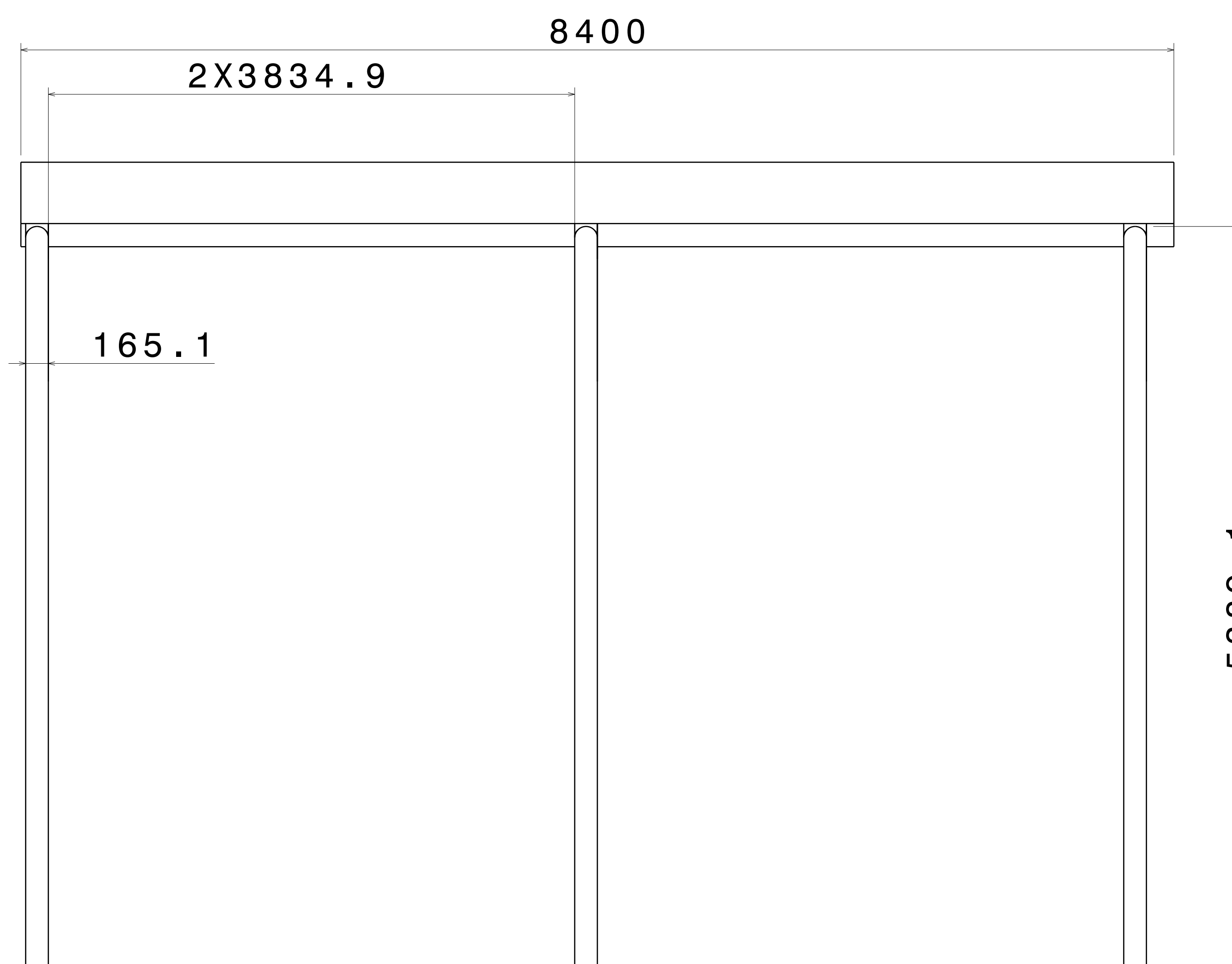
RIGHT VIEW SCALE: 1:25
