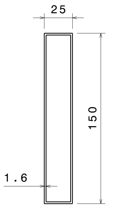
Right view Scale: 1:2
