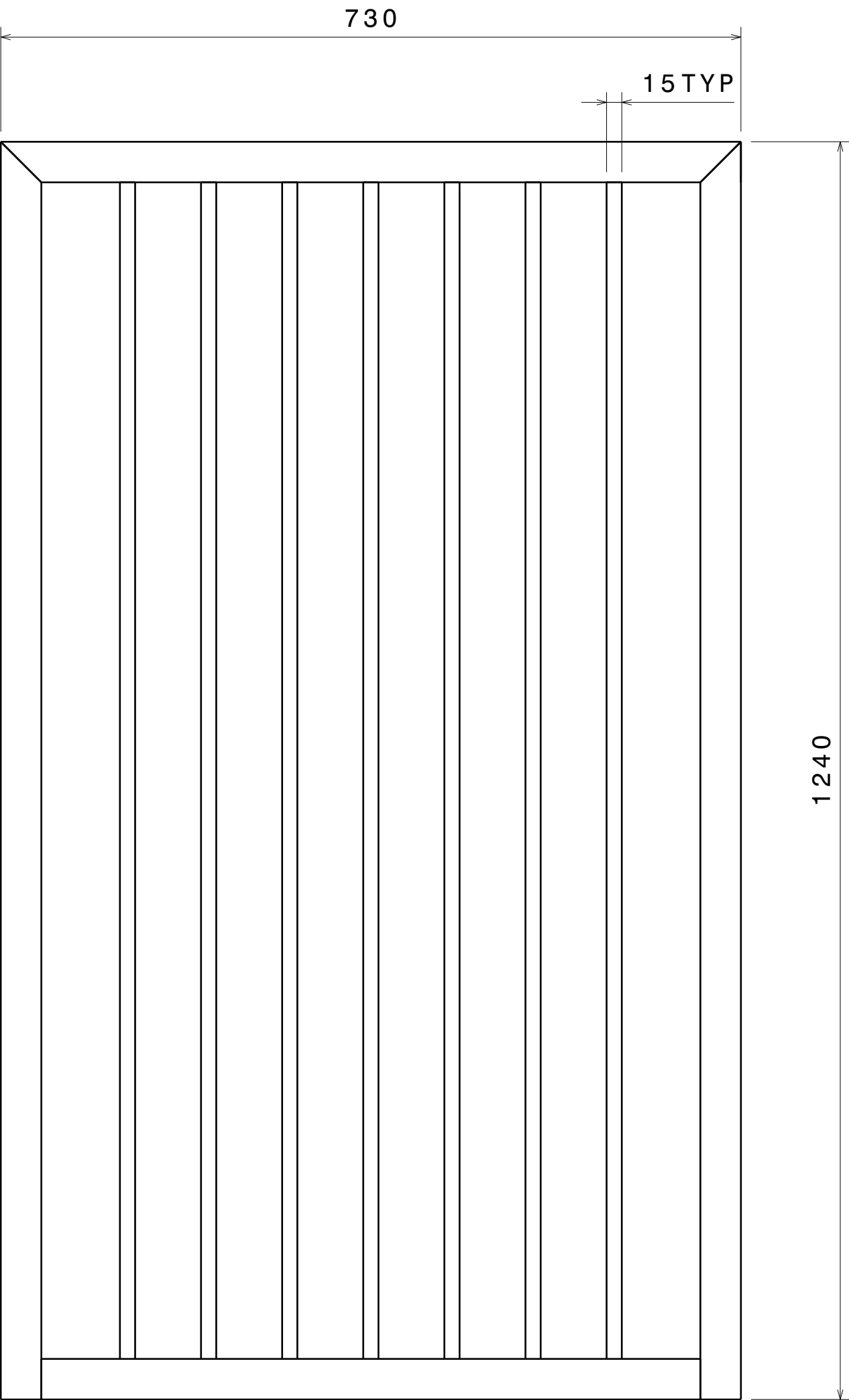
Right view Scale: 1:5
