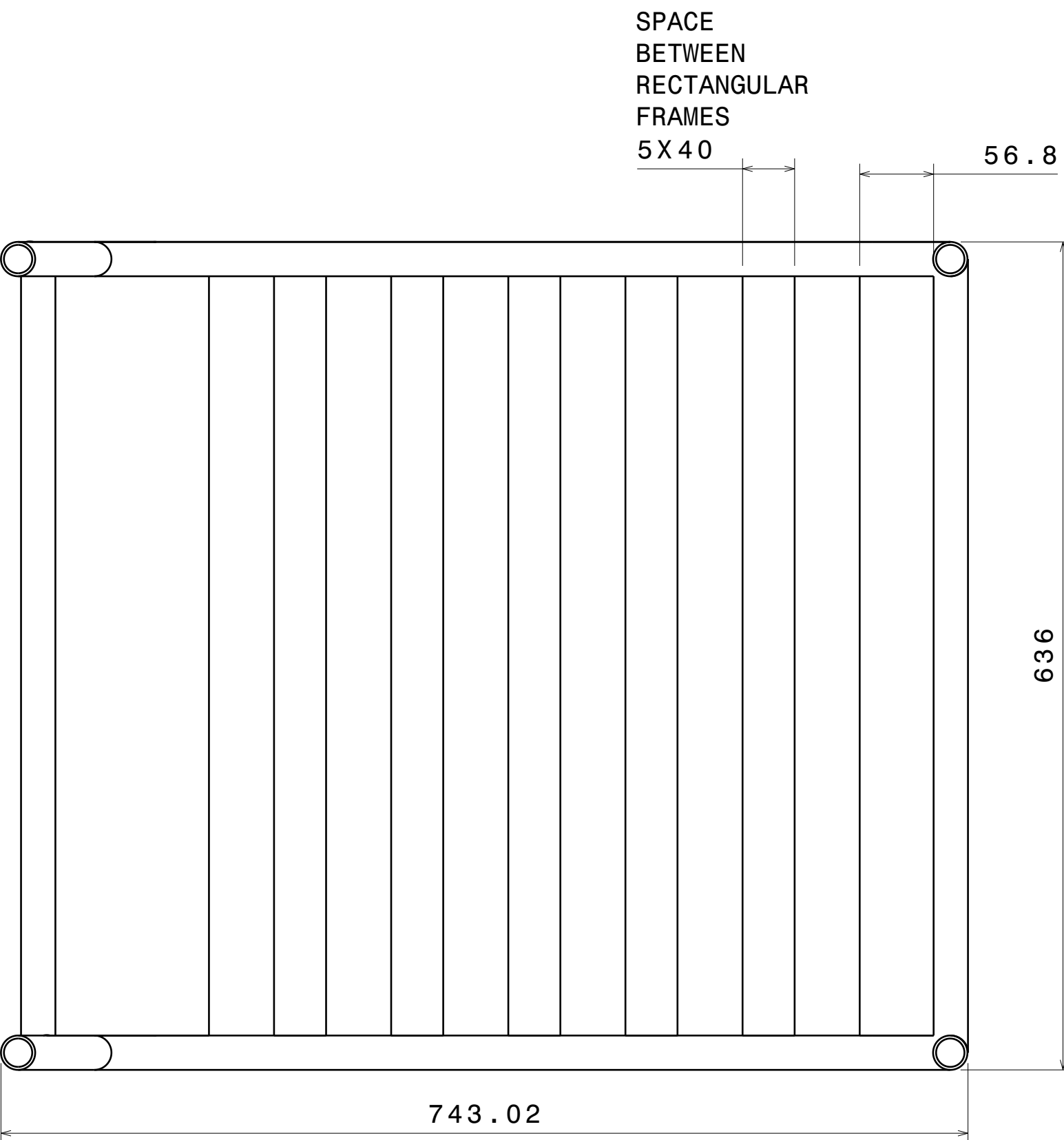
Bottom view[2] Scale: 1:4
