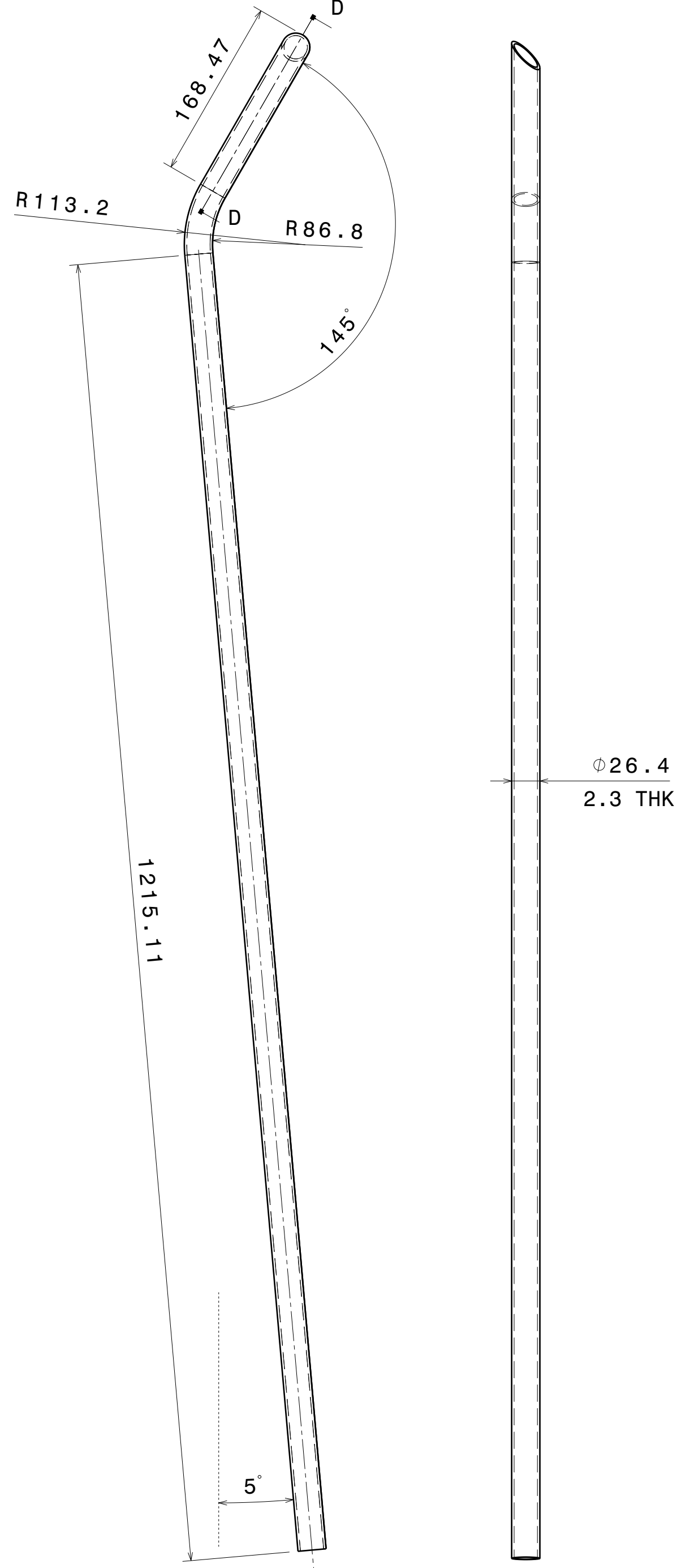
Right view[3] Scale: 1:4
