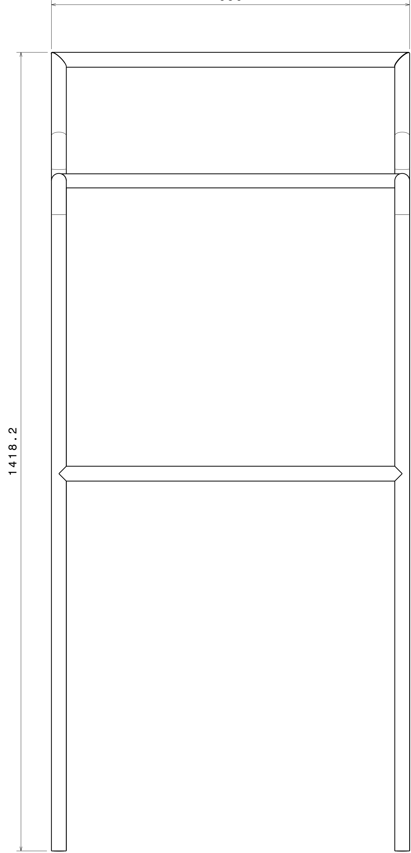
Right view[2] Scale: 1:4
