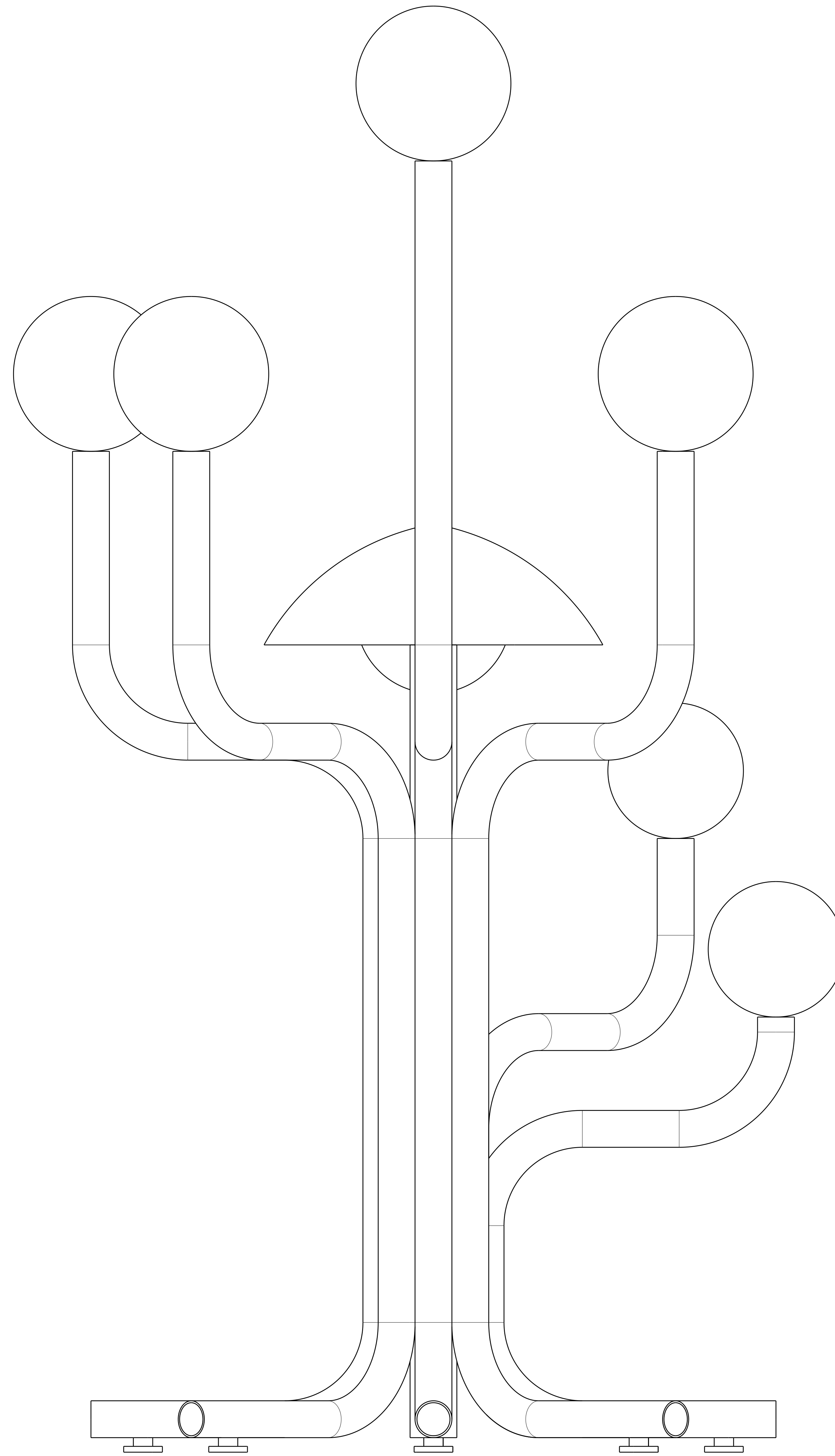
Right view Scale: 2:5
