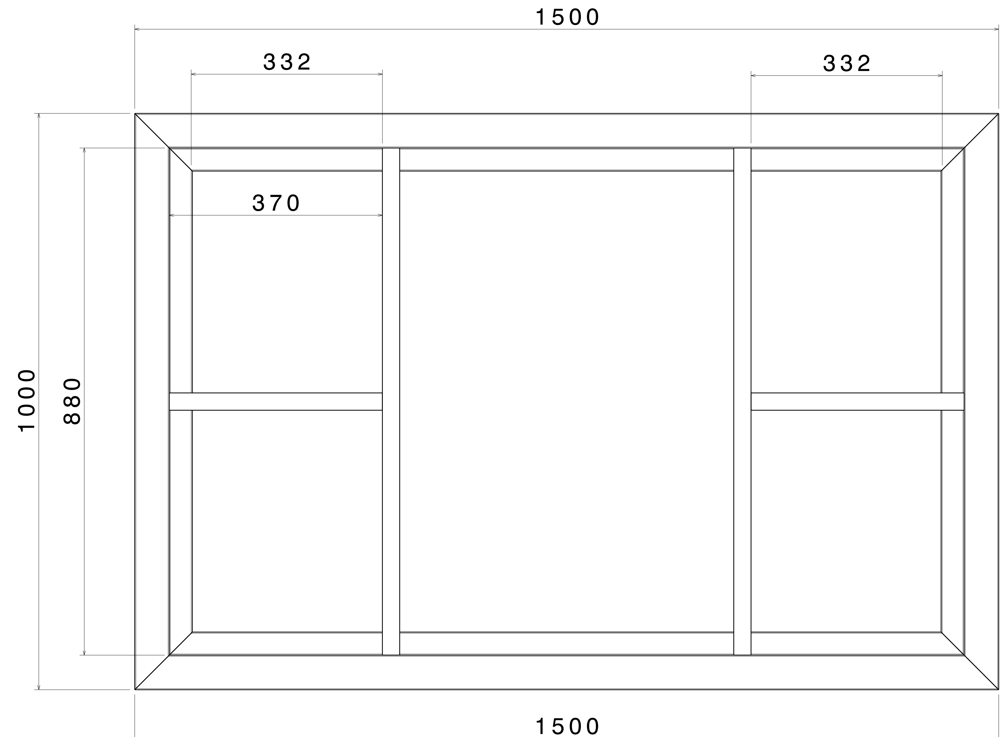
Front view Scale: 1:4
