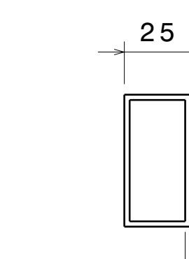
Right view Scale: 1:2
