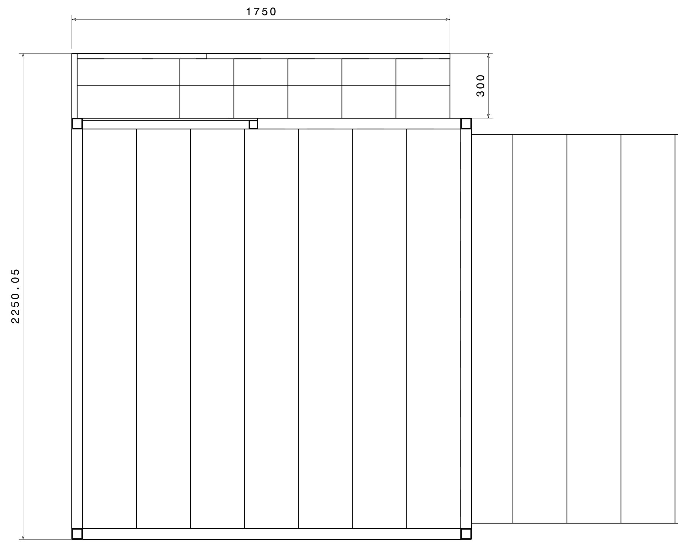
Top view Scale: 1:10
