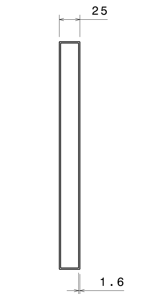
Right view[2] Scale: 7:20
