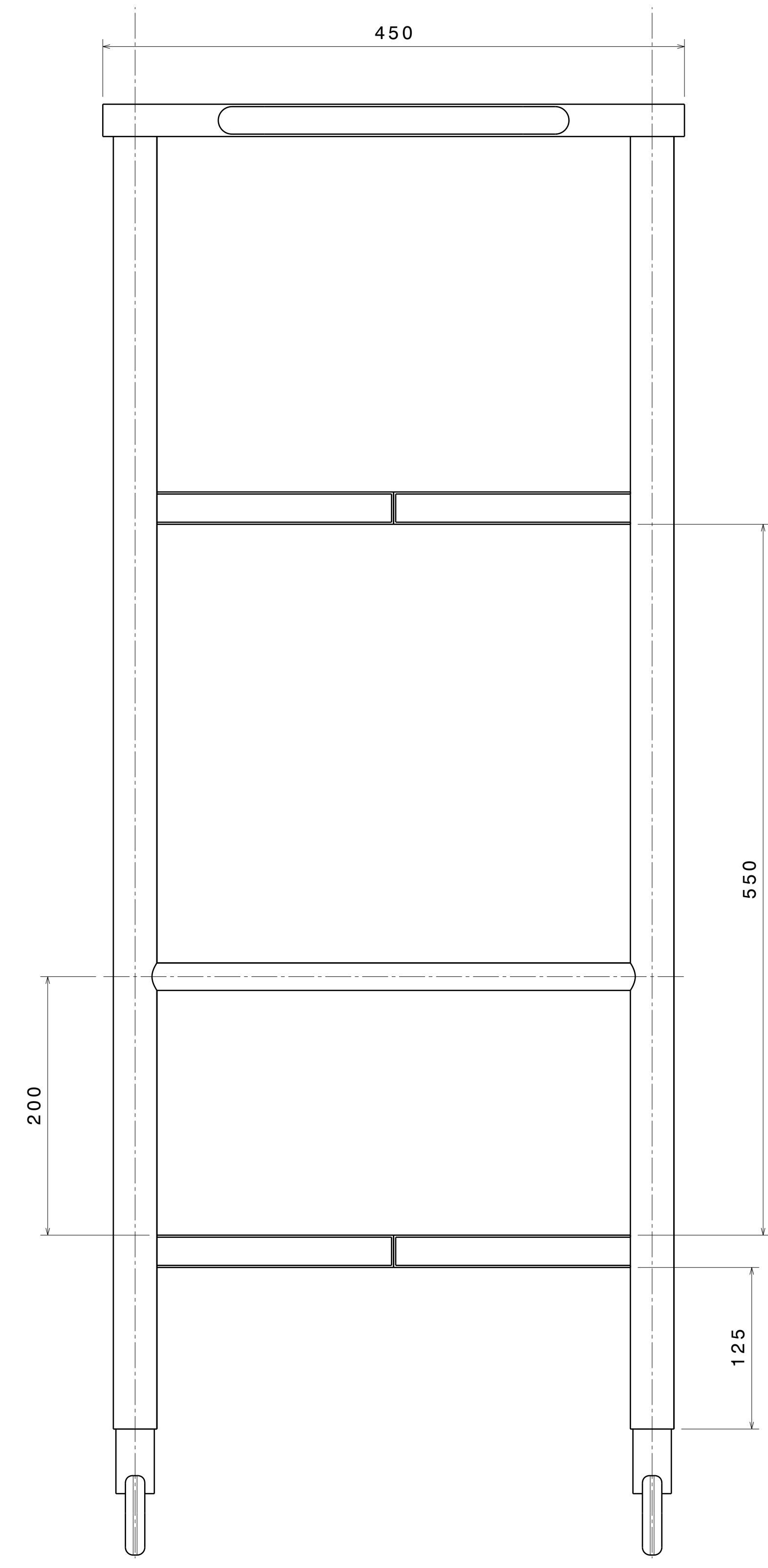
Right view Scale: 7:20
