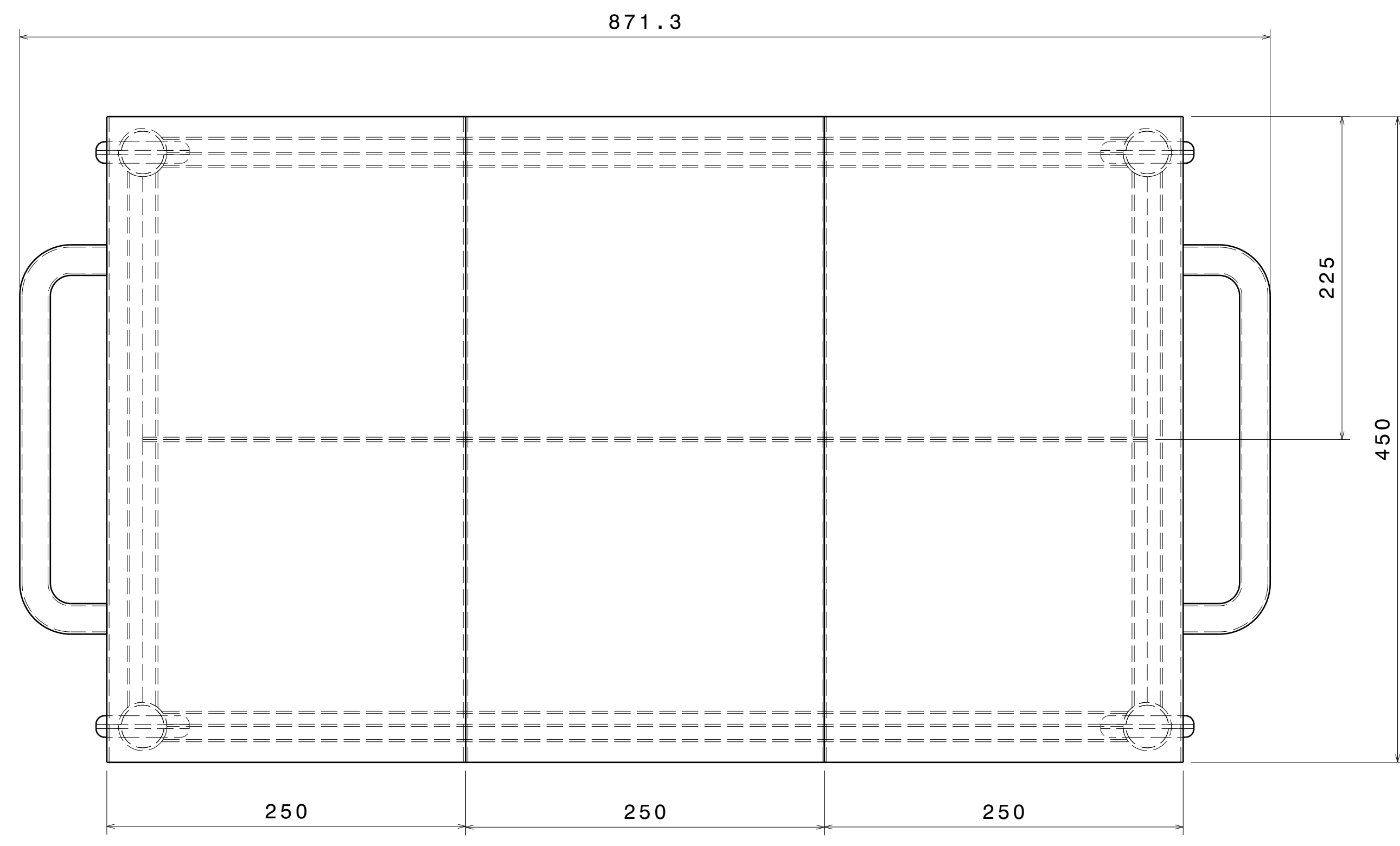
Top view Scale: 7:20
