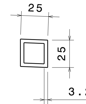
Right view Scale: 1:2
