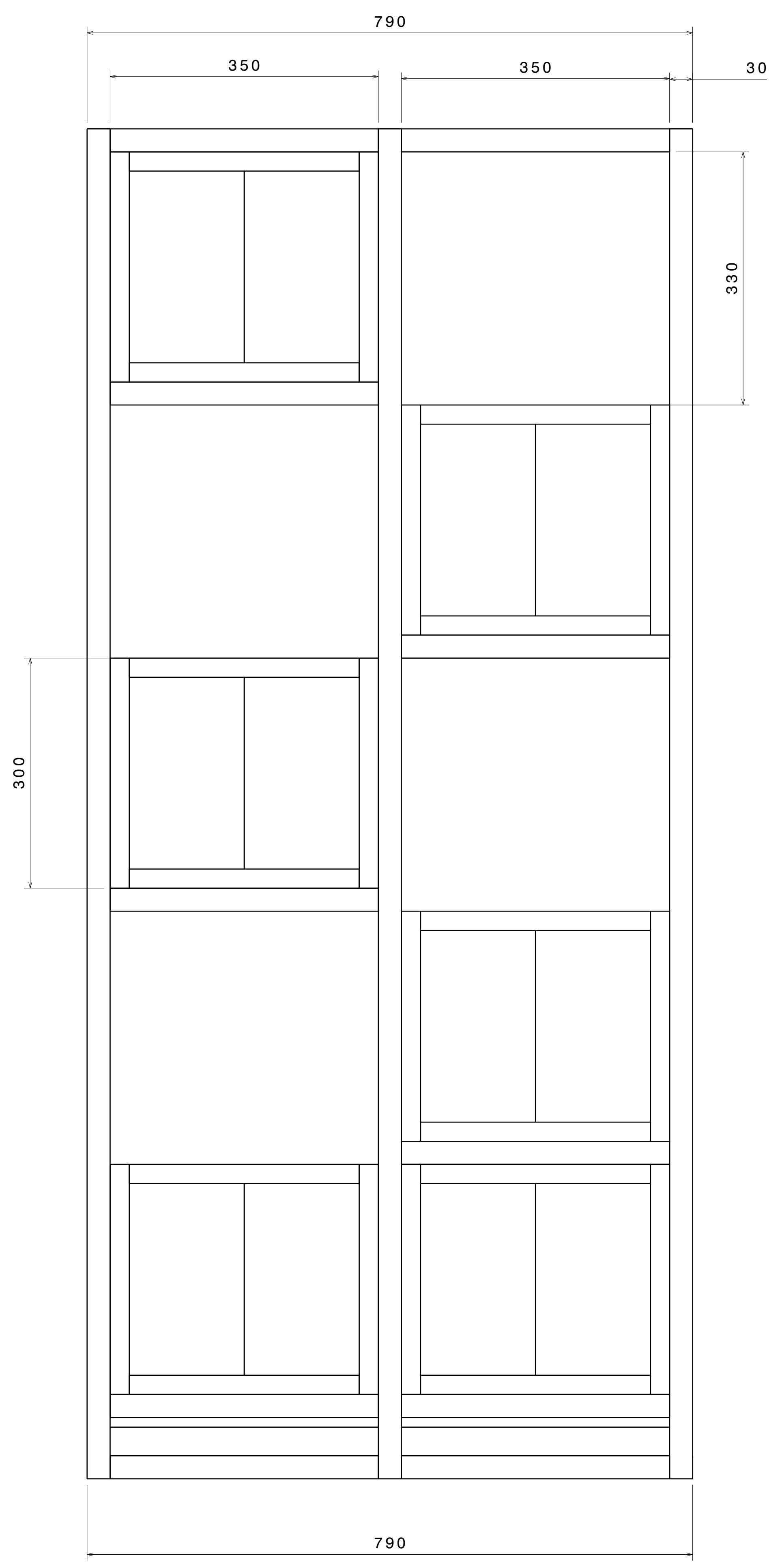
Right view Scale: 1:4
