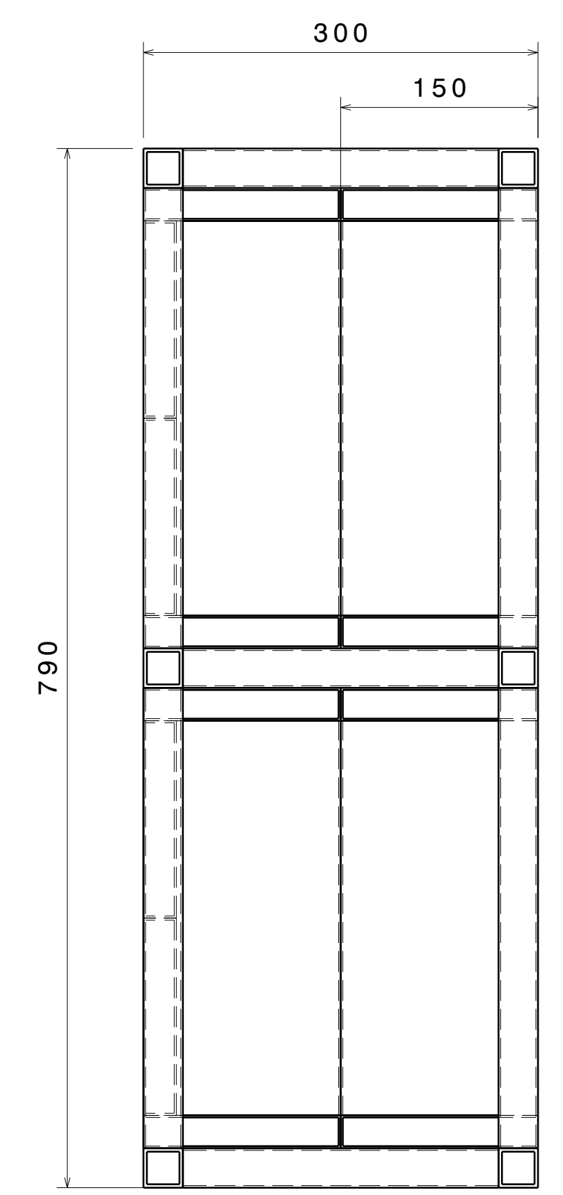
Top view Scale: 1:4
