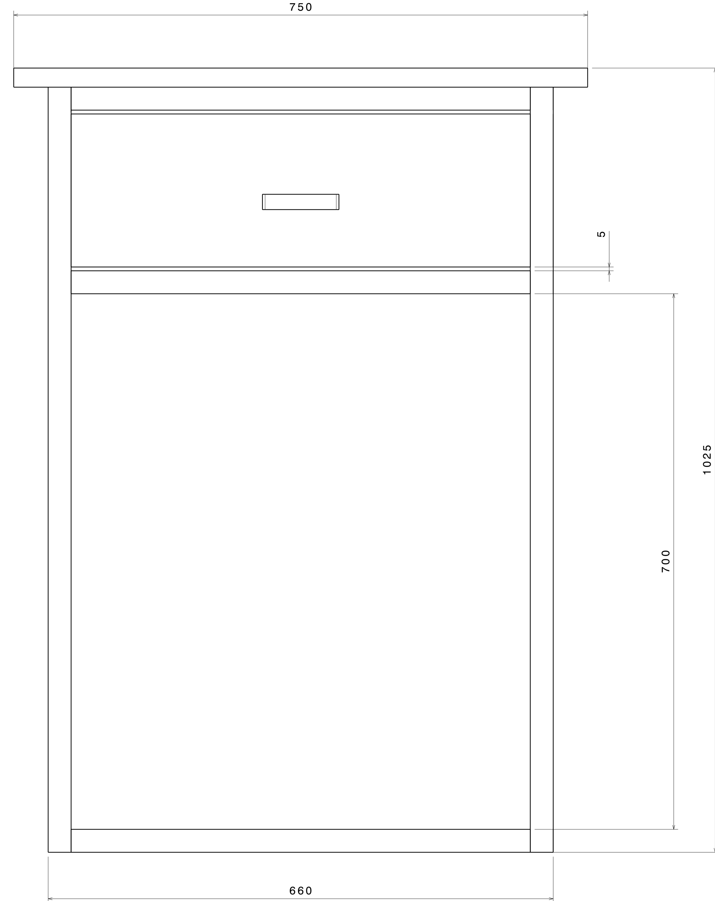
Right view Scale: 7:20
