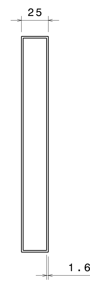
Right view Scale: 1:2
