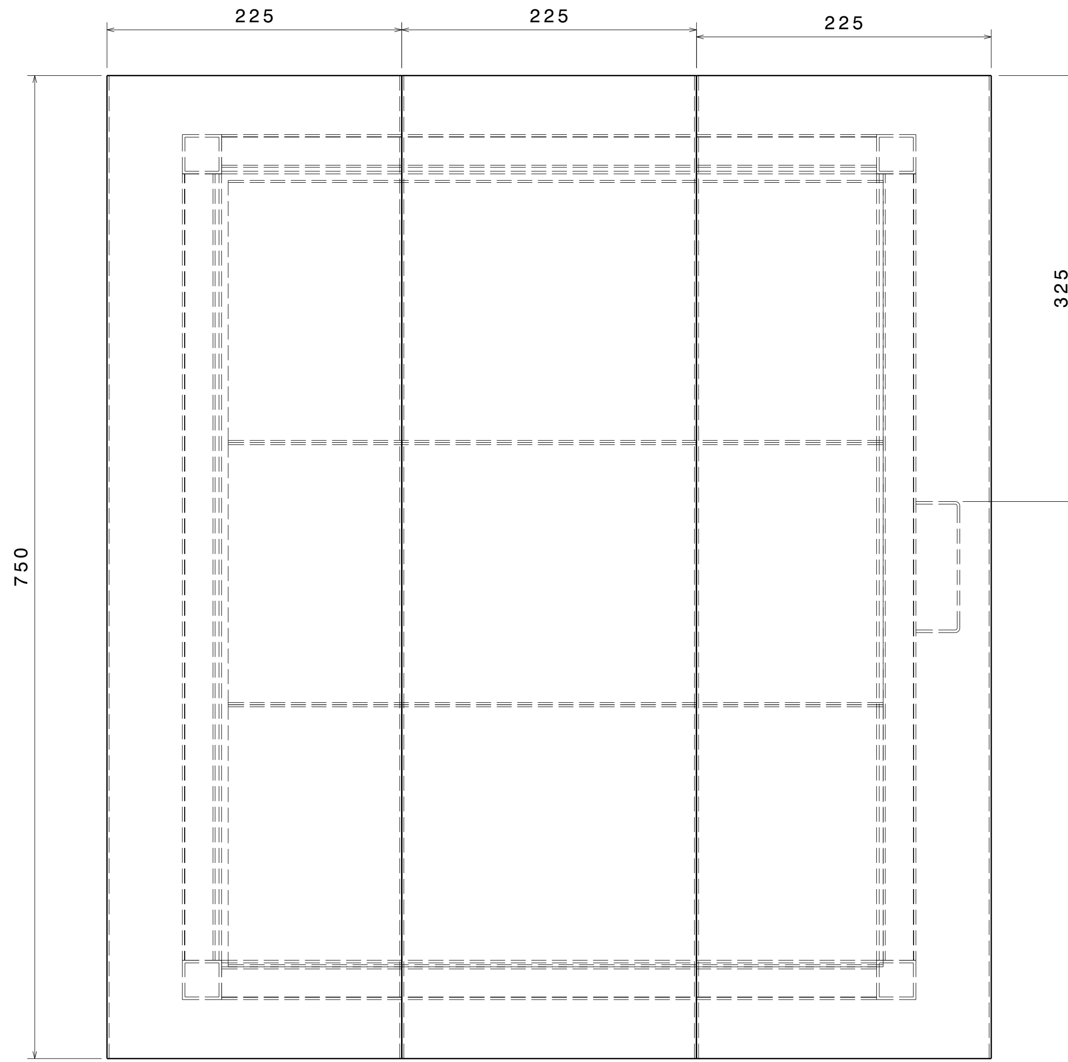
Top view Scale: 7:20
