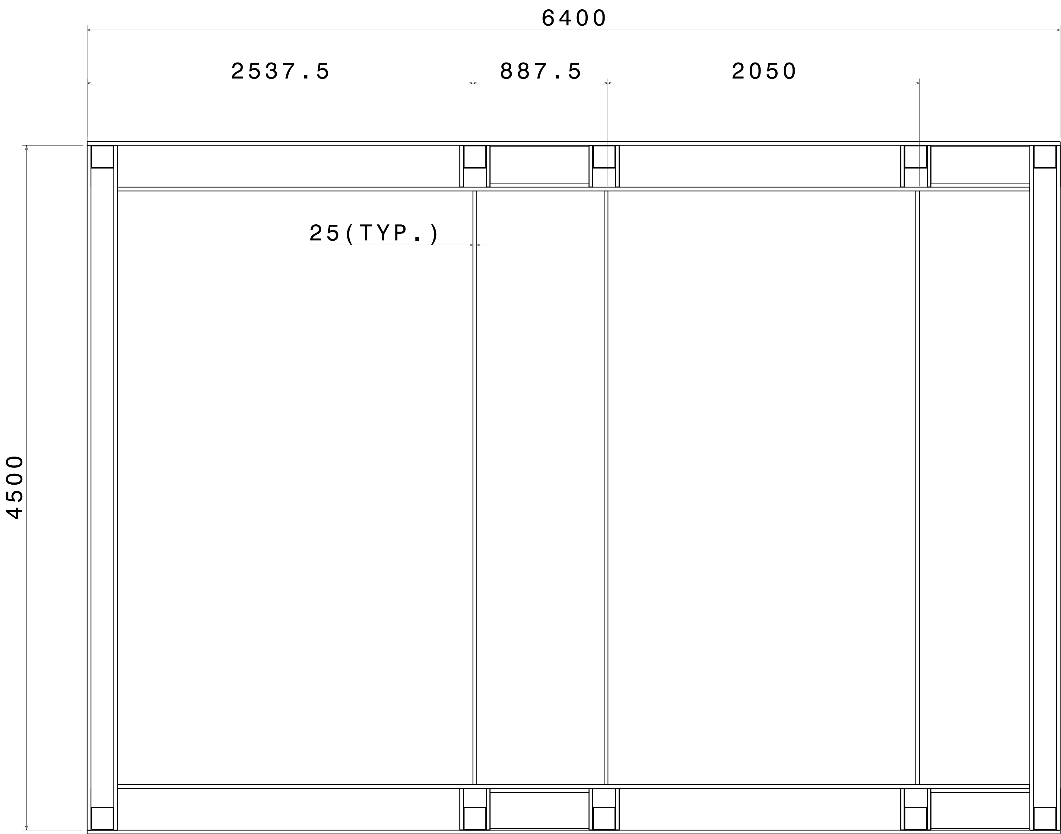
FRONT VIEW SCALE: 1:5
