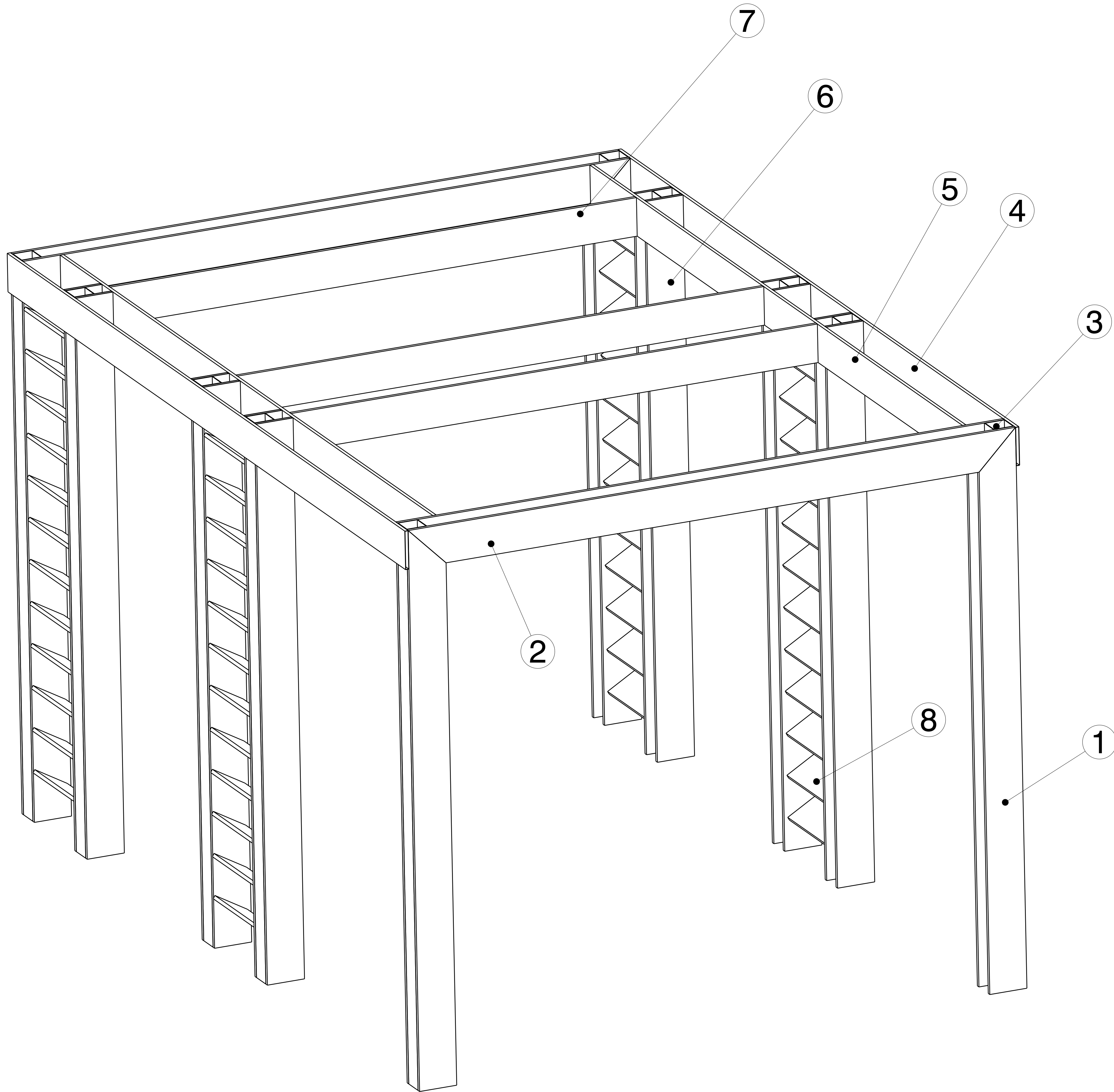
ISOMETRIC VIEW SCALE: 1:15
