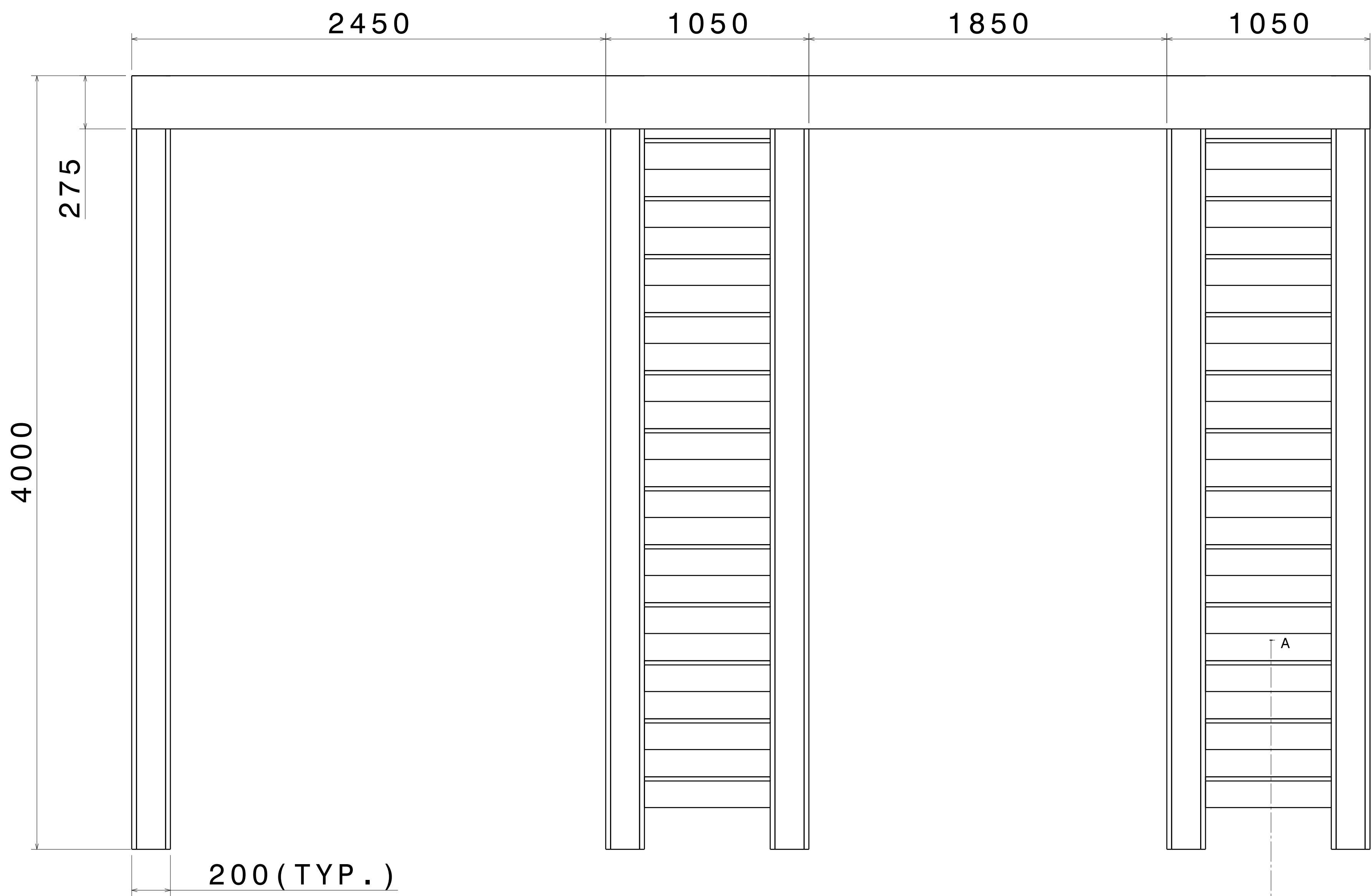
BOTTOM VIEW SCALE: 1:5
