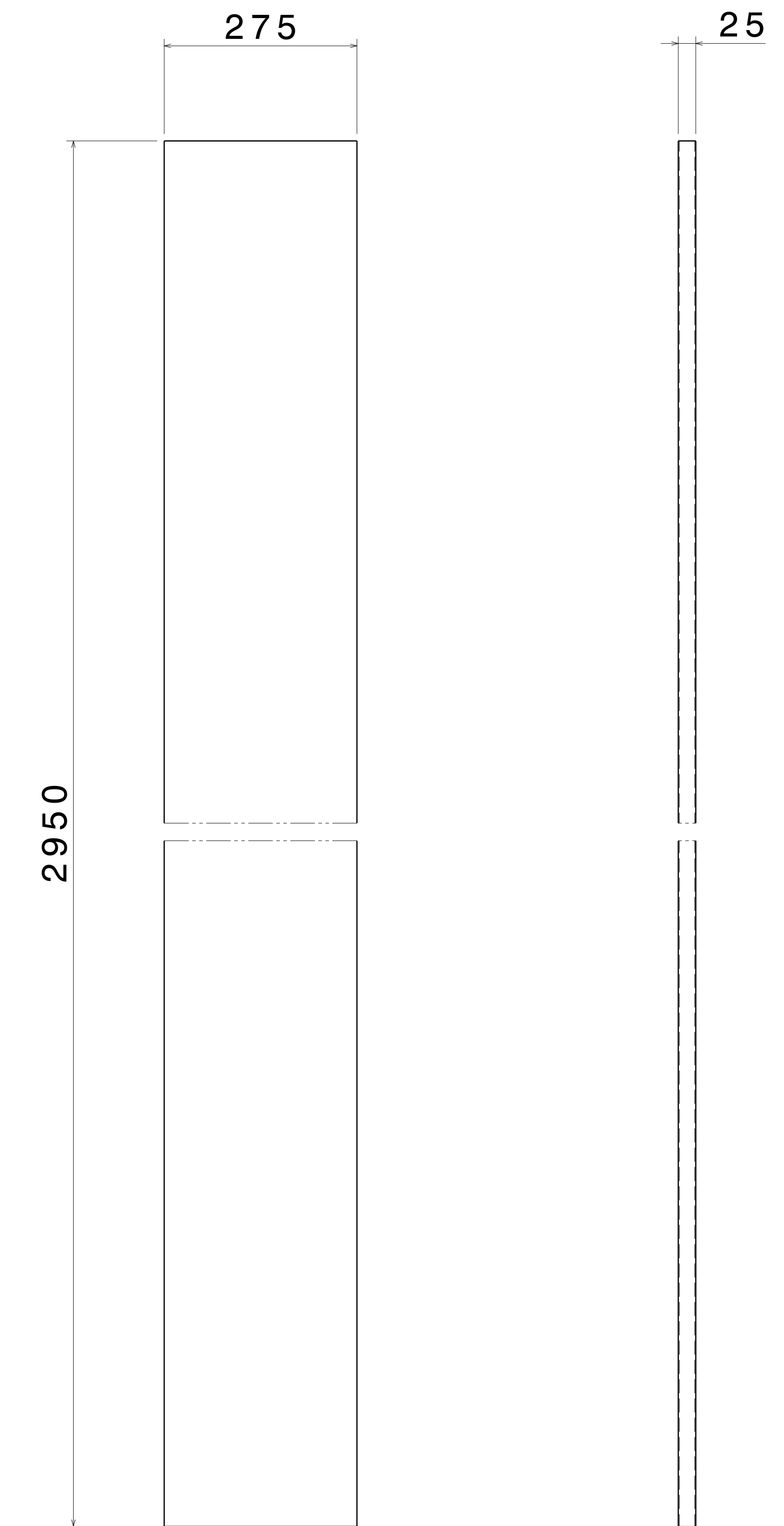
FRONT VIEW SCALE: 1:5 RIGHT VIEW SCALE: 1:5
