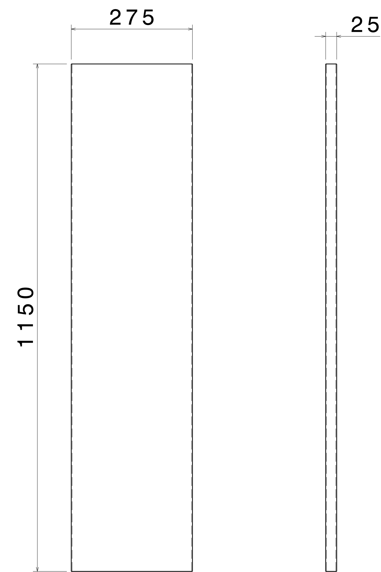
FRONT VIEW SCALE: 1:5 RIGHT VIEW SCALE: 1:5
