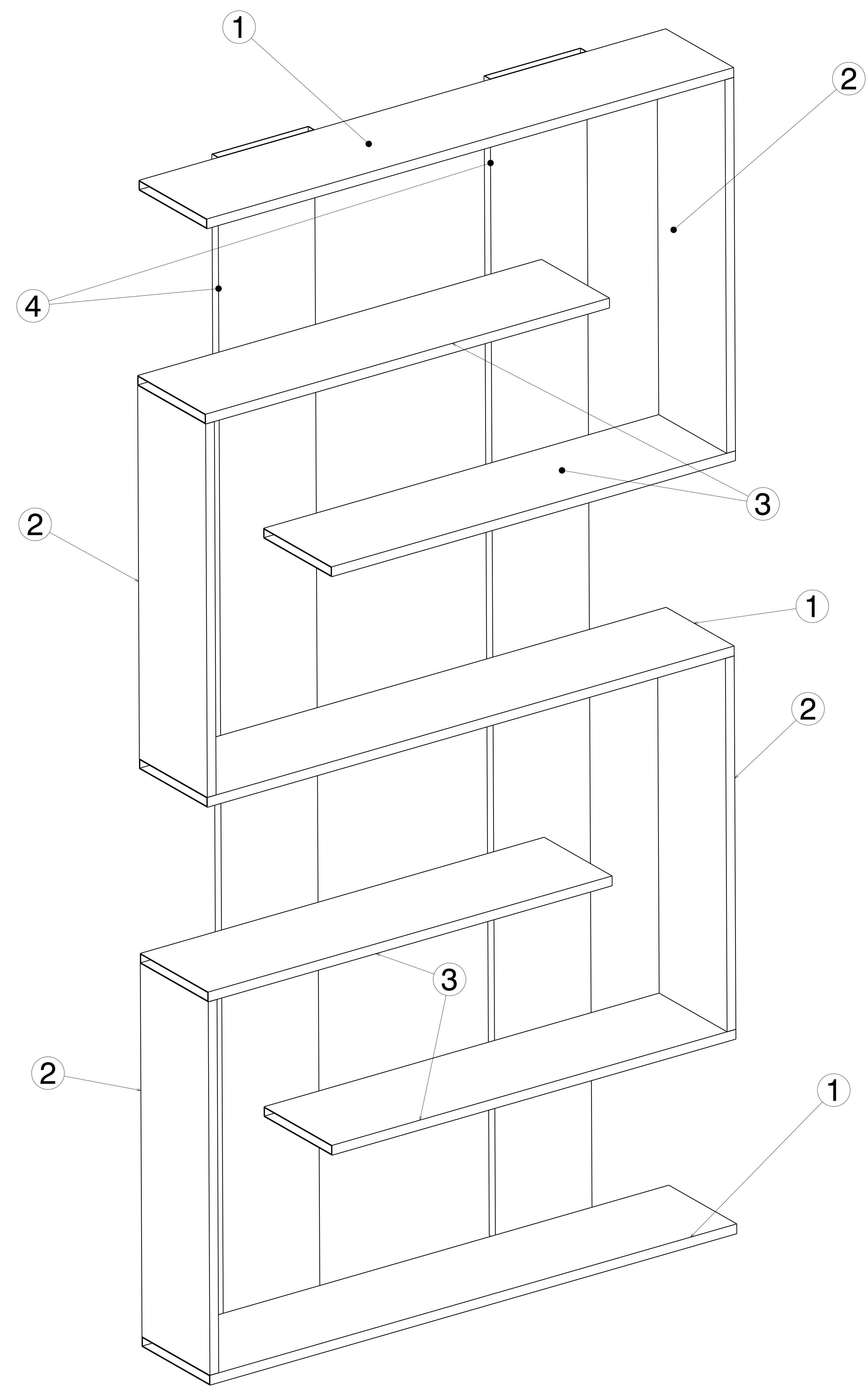
ISOMETRIC VIEW SCALE: 1:5
