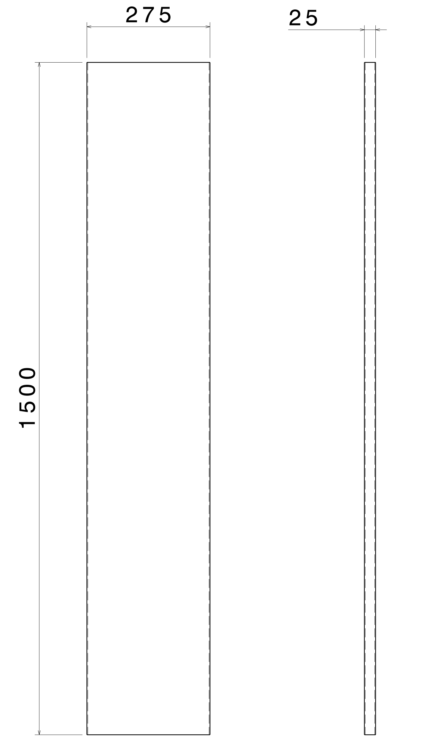
FRONT VIEW SCALE: 1:5 RIGHT VIEW SCALE: 1:5
