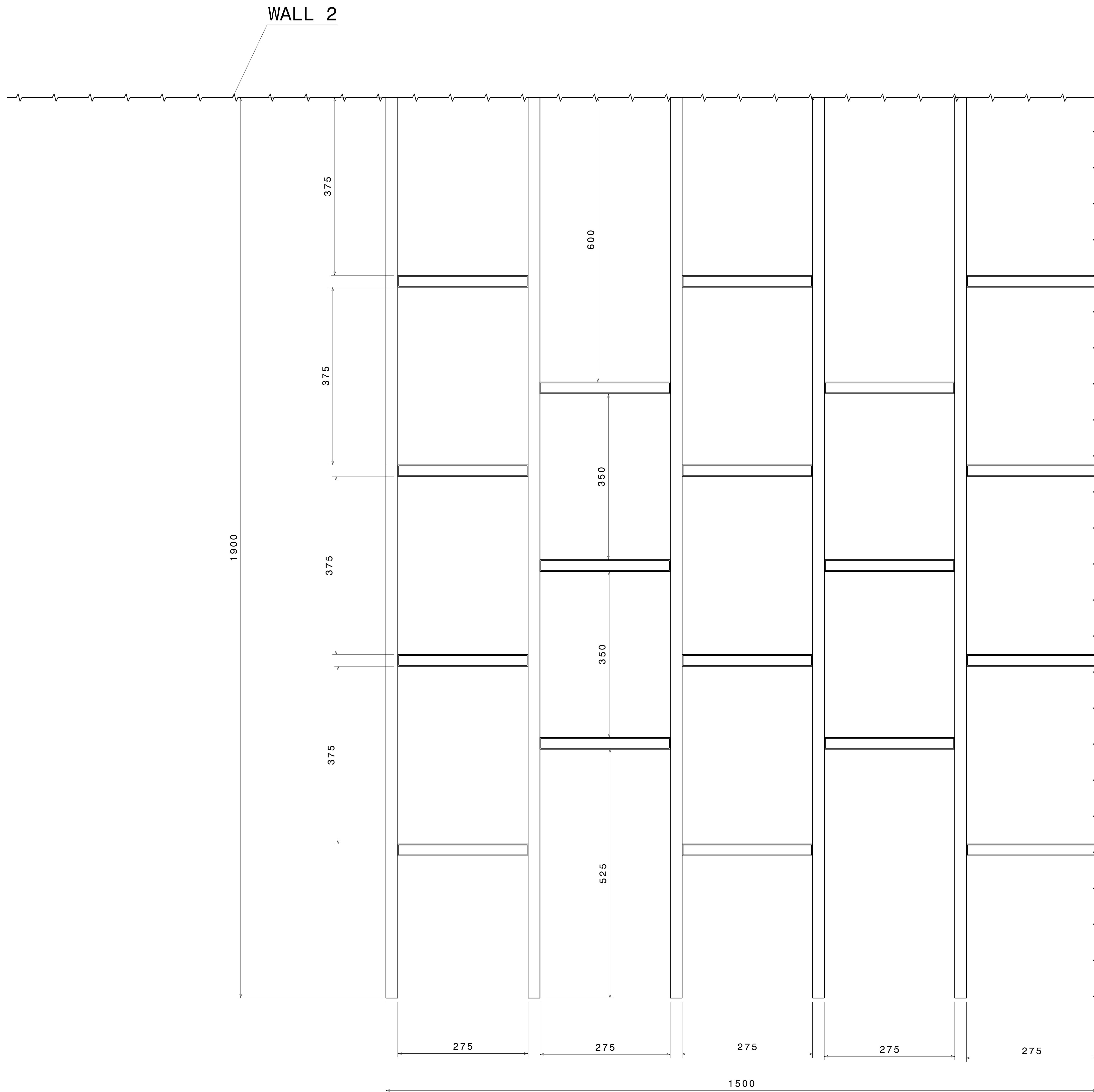
Front view Scale: 1:4
