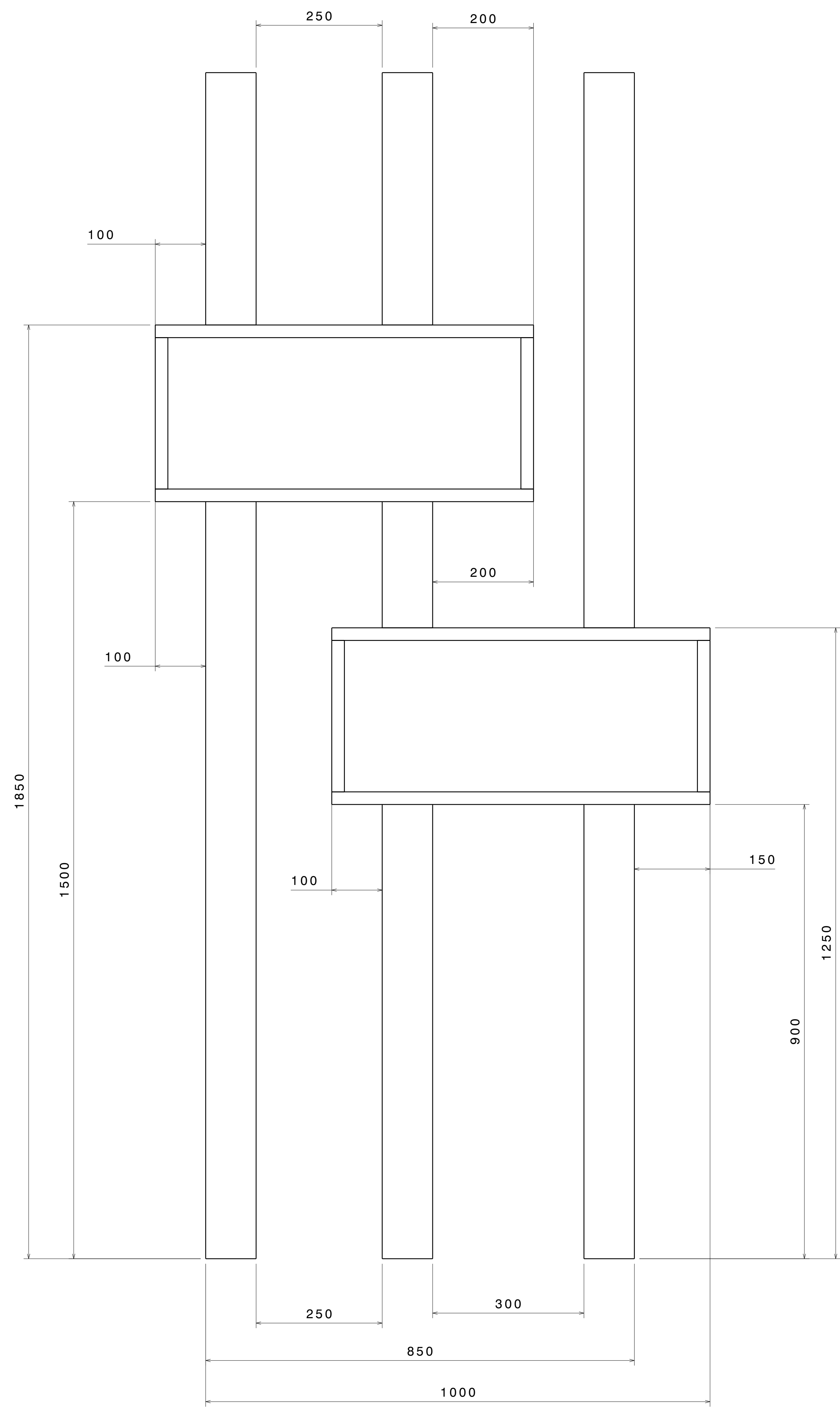
Front view Scale: 1:5
