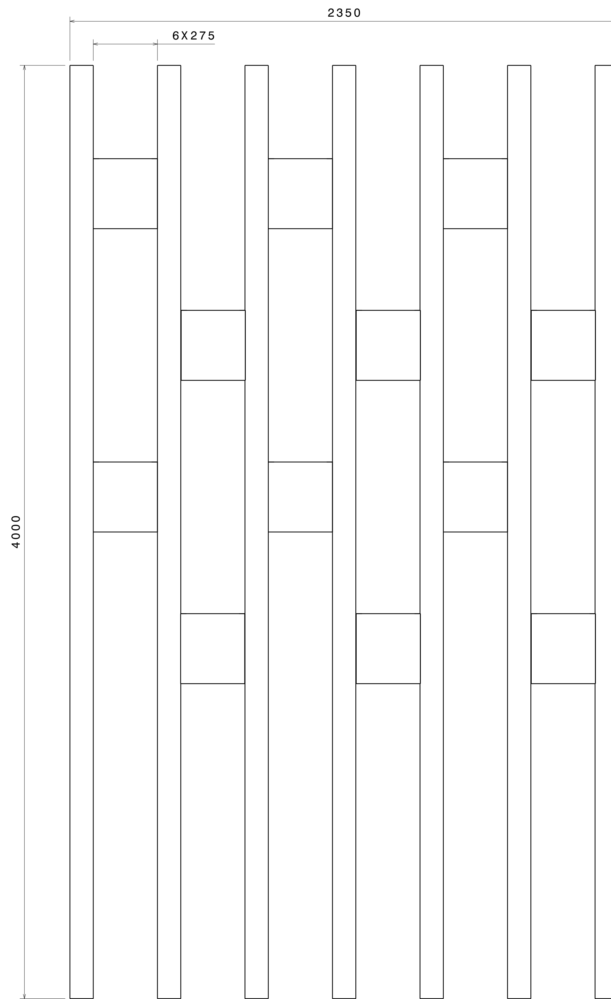
Top view Scale: 1:10
