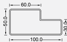
SINGLE DOOR FRAME - 100 x 50
