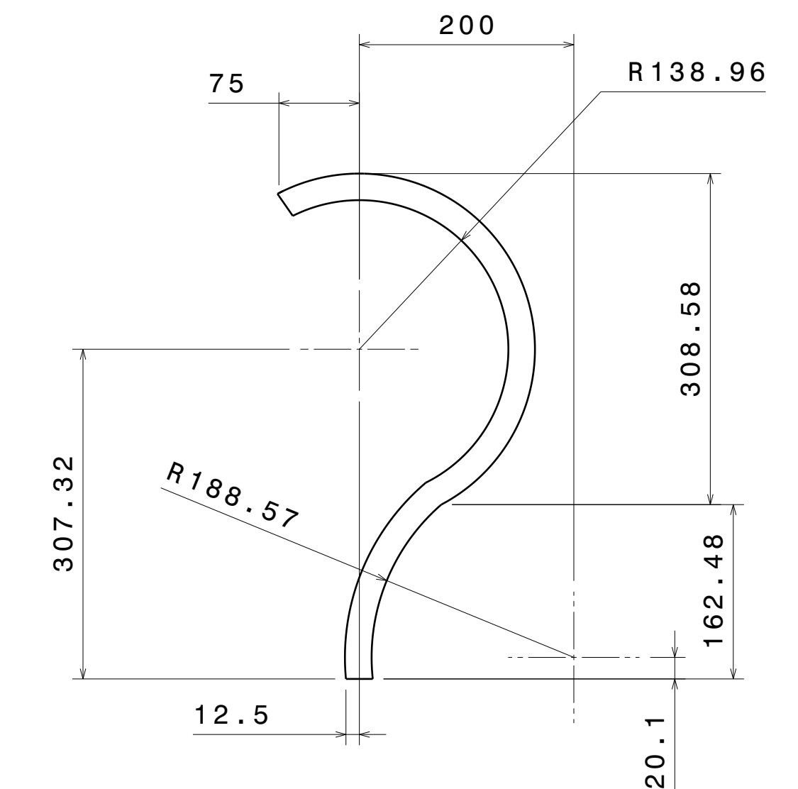
ITEM 14 SECTION: 25X25X1.6
