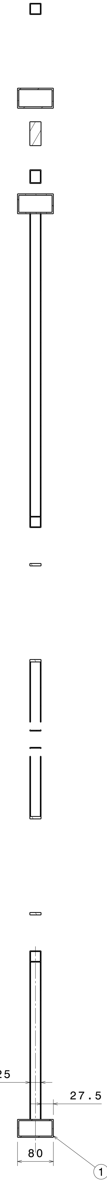
Section cut B-B Scale: 1:5
