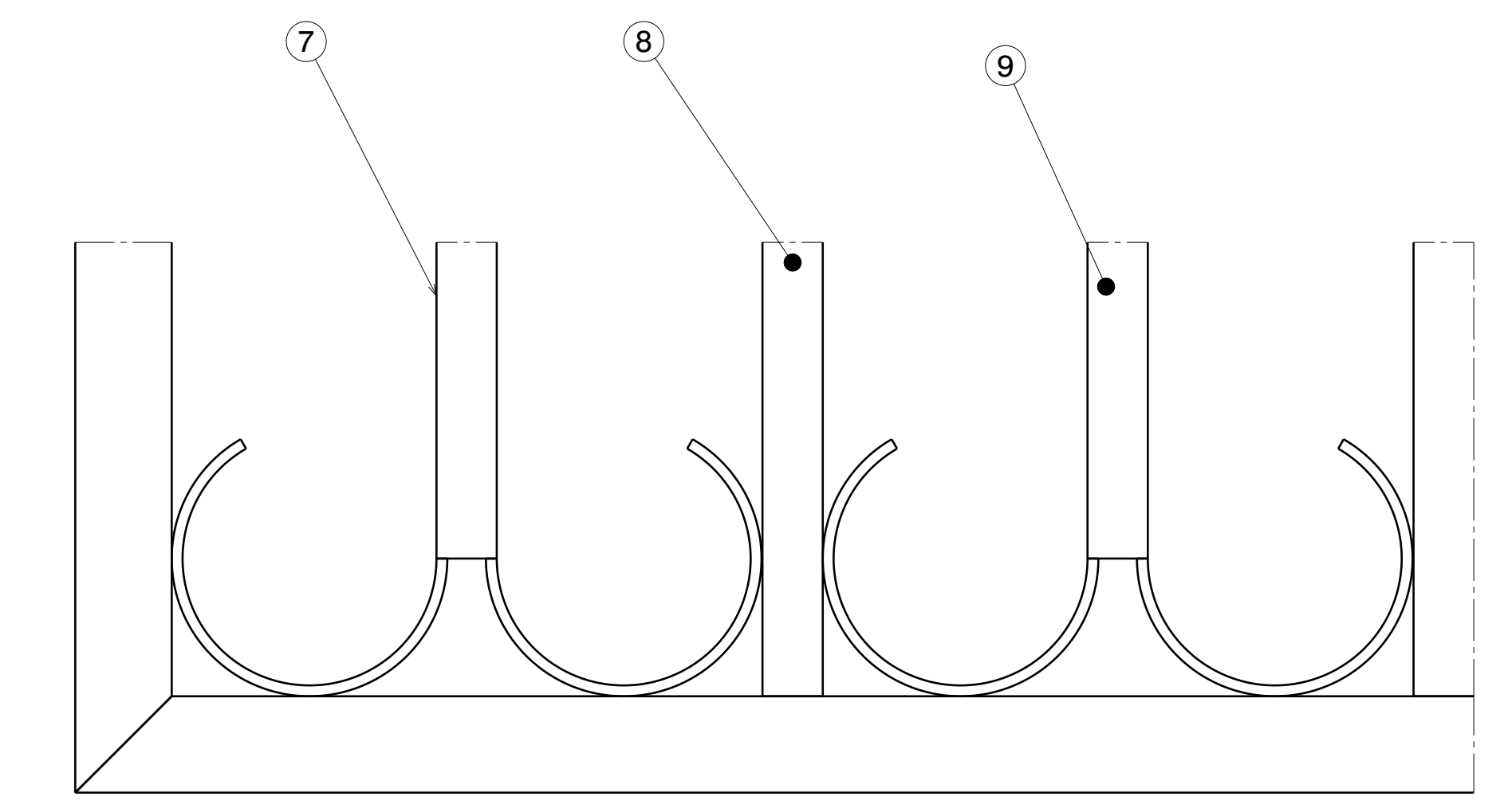
Detail C Scale: 2:5
