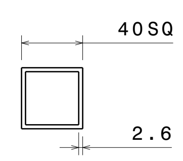
Right view Scale: 2:5
