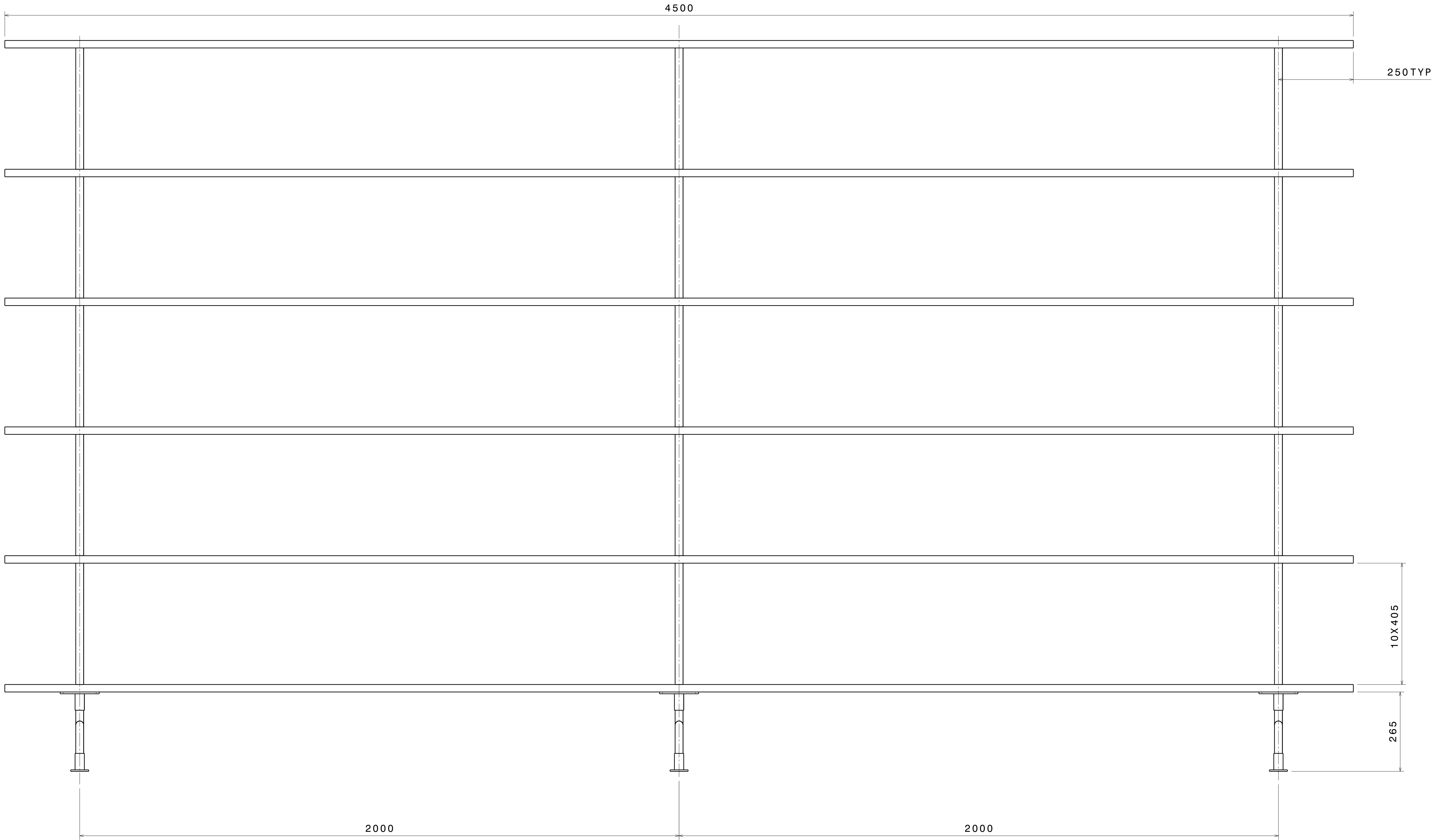
Front view Scale: 3:20
