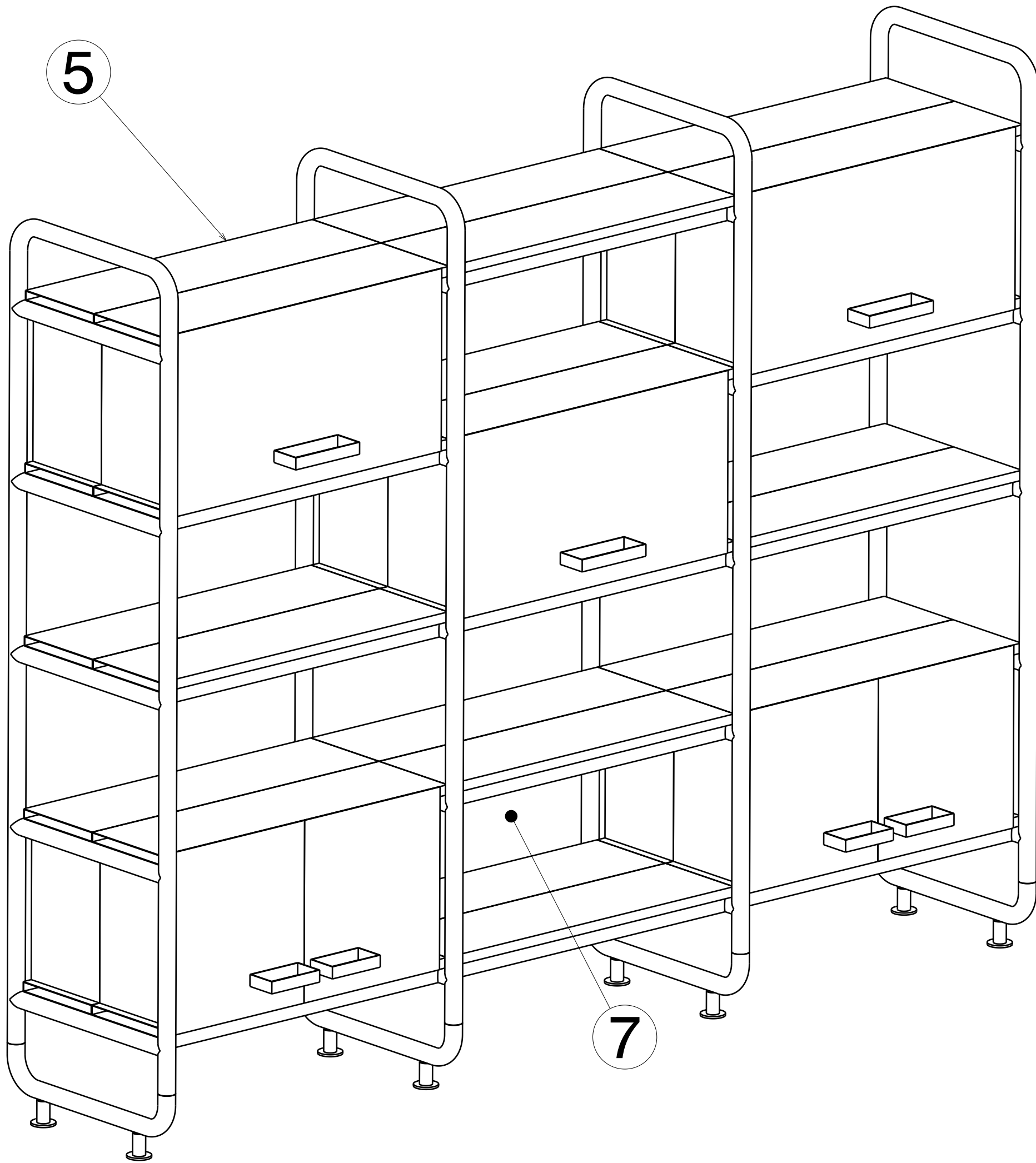
Isometric view Scale: 1:10
