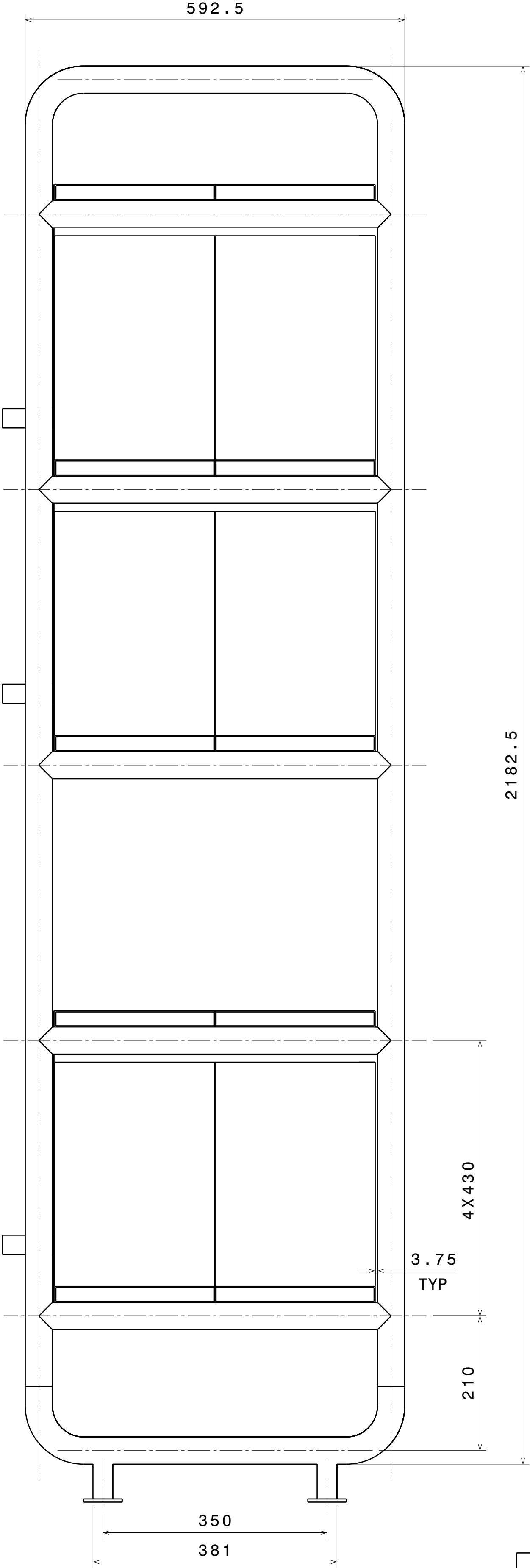
Right view Scale: 1:5
