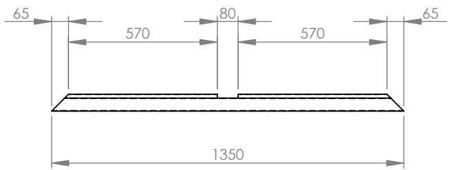
ITEM 4 DDF 130X65X2.0X1350 (2)
