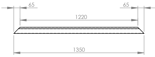
ITEM 2 DDF 130X65X2.0X1350
