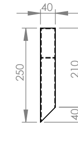
ITEM 6 RHS 80X40X2.0X250 (3)
