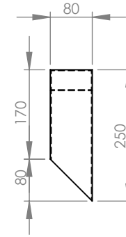
ITEM 3 RHS 80X40X2.0X250 (2)
