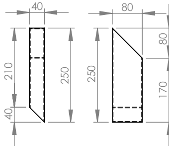
ITEM 5 RHS 80X40X2.0X250 (4)
