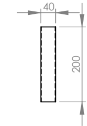
ITEM 4 RHS 80X40X2.0X200
