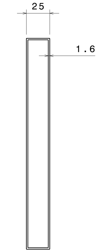
Right view Scale: 1:2
