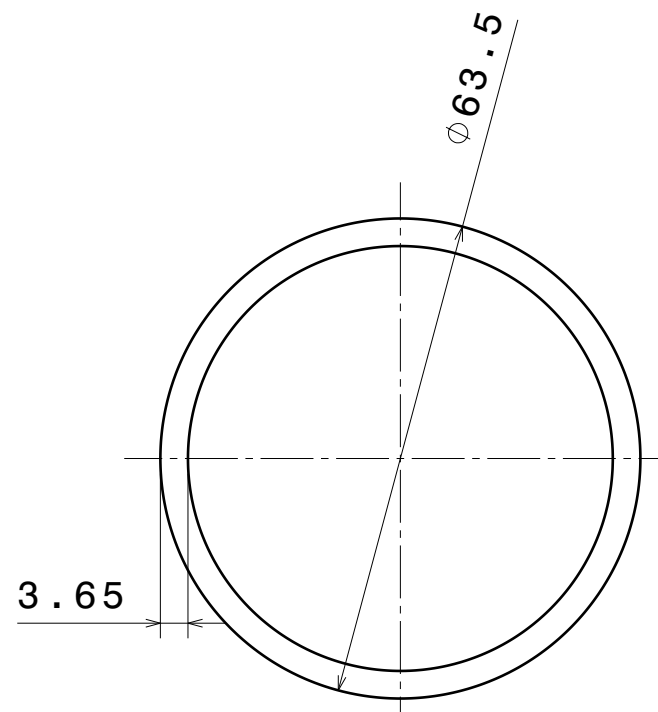
Right view[2] Scale: 1:1
