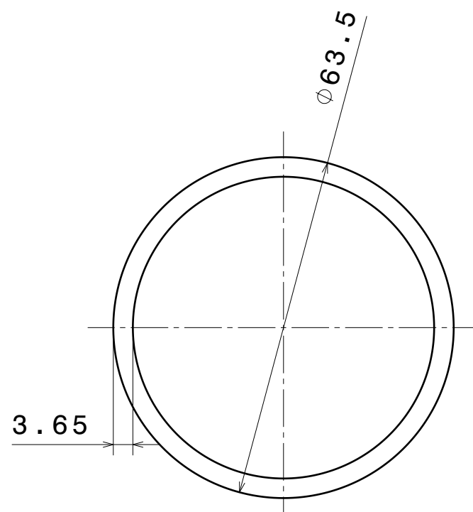
Right view[3] Scale: 1:1
