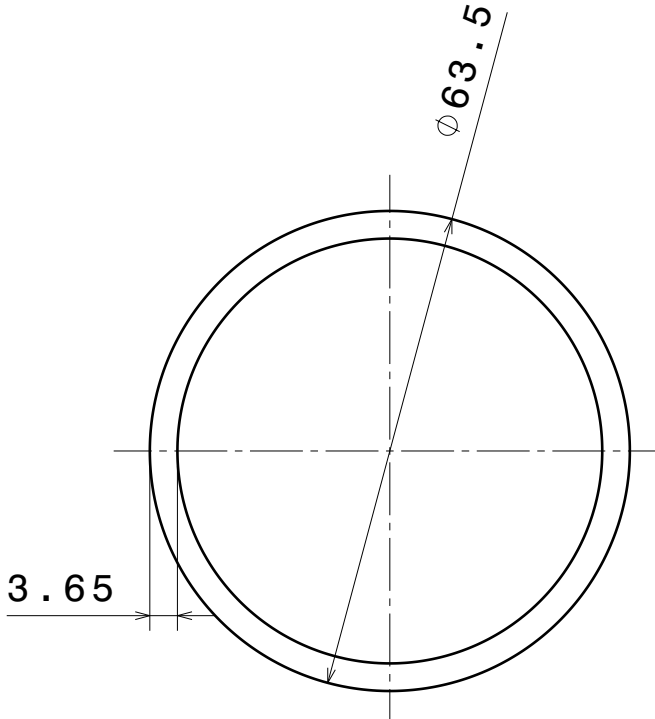
Right view Scale: 1:1
