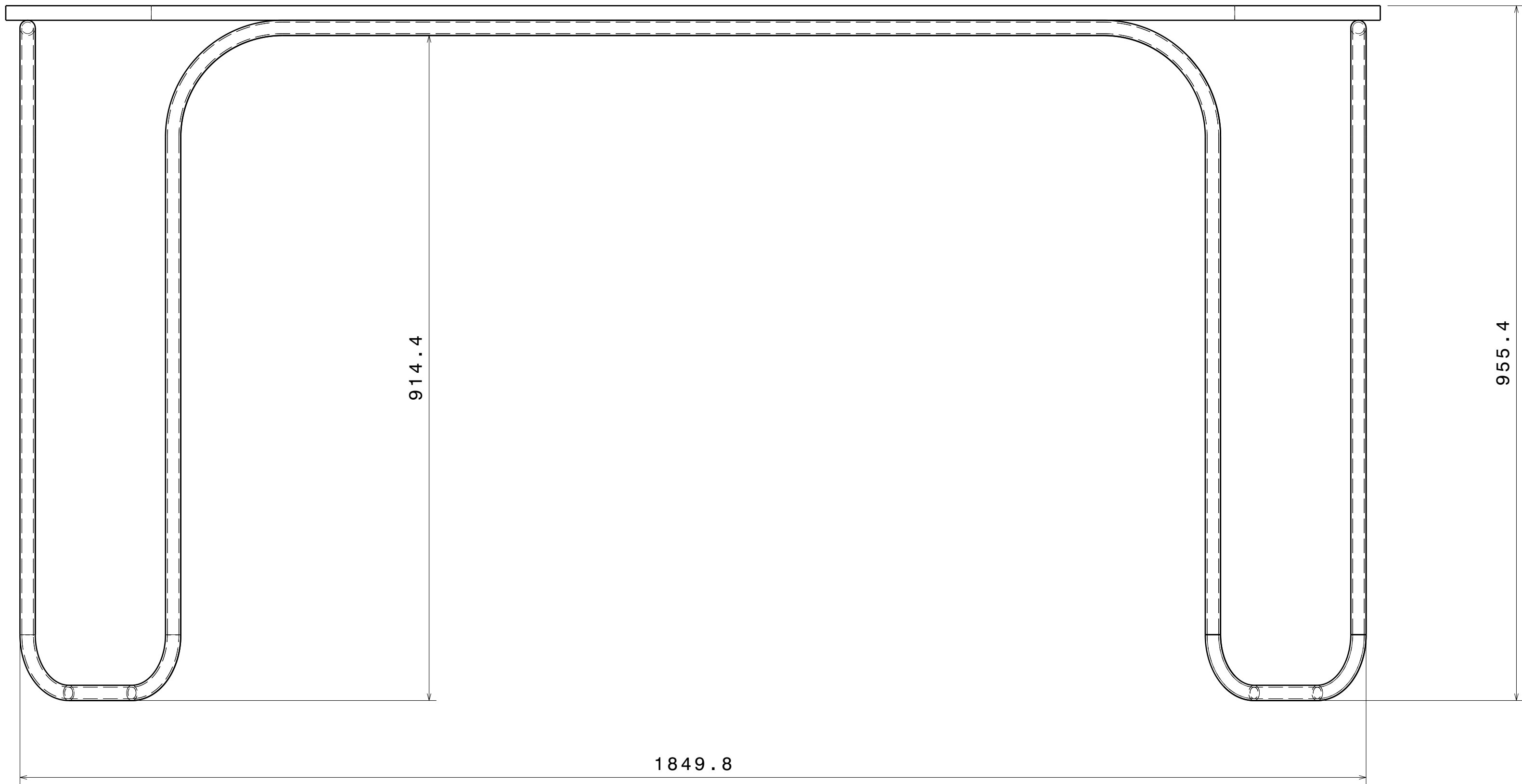
Bottom view Scale: 1:5
