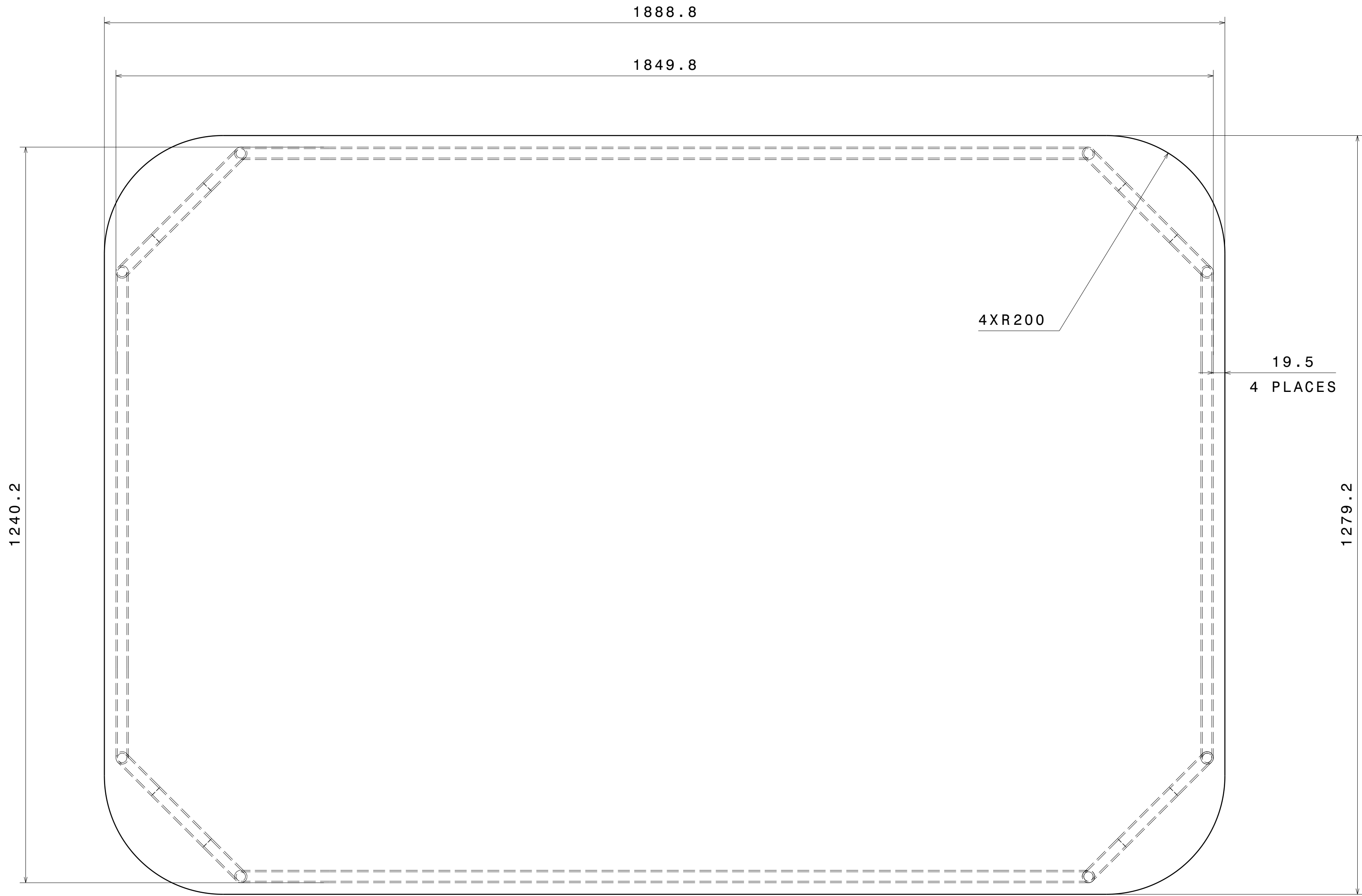
Front view Scale: 1:5
