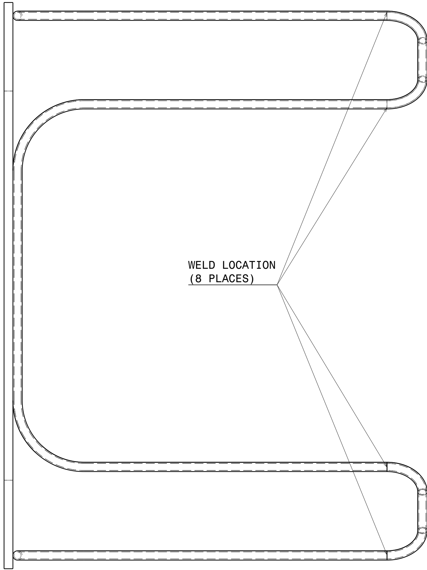
Right view Scale: 1:5
